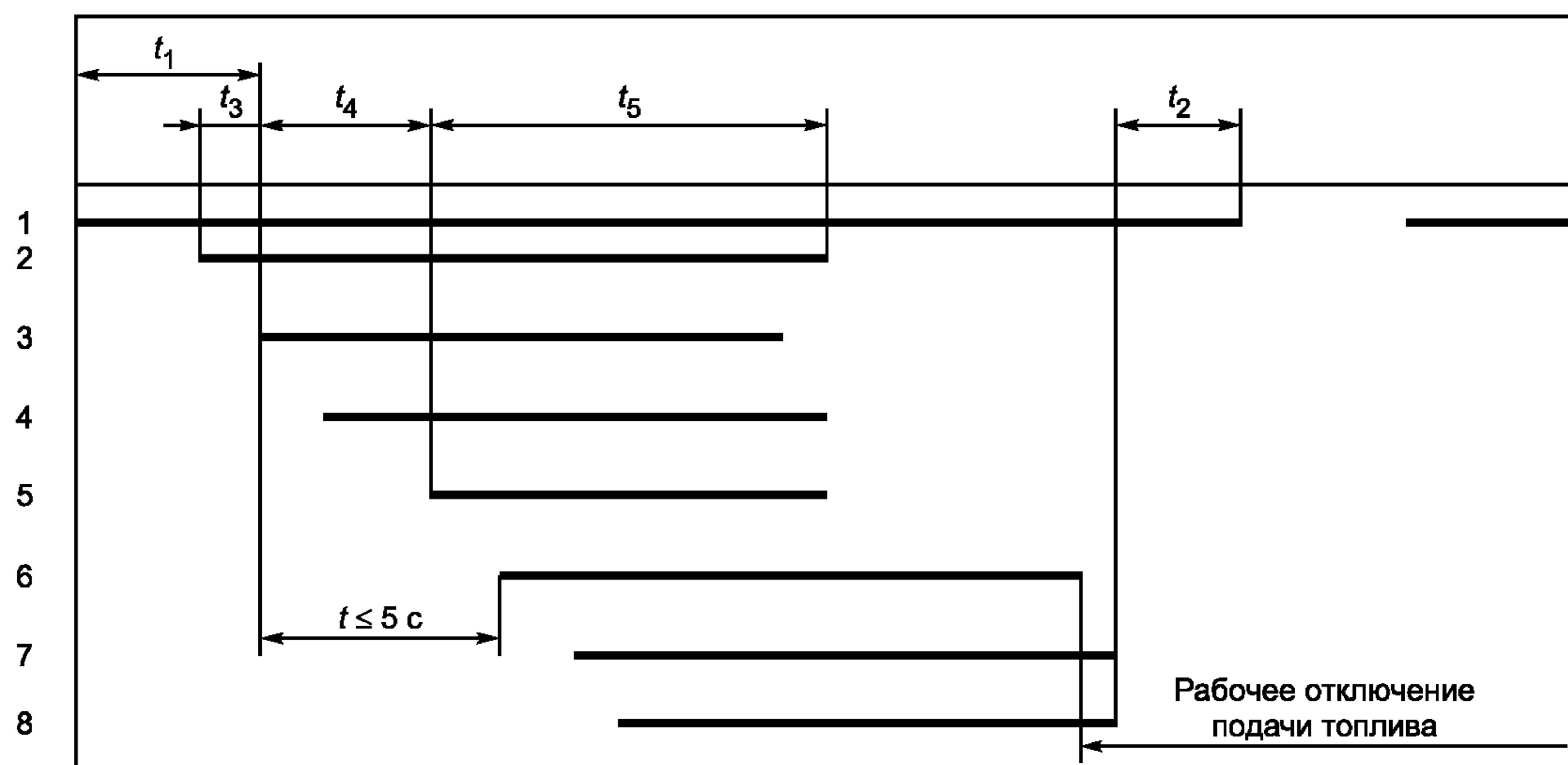
Диаграмма нормальной работы горелки
