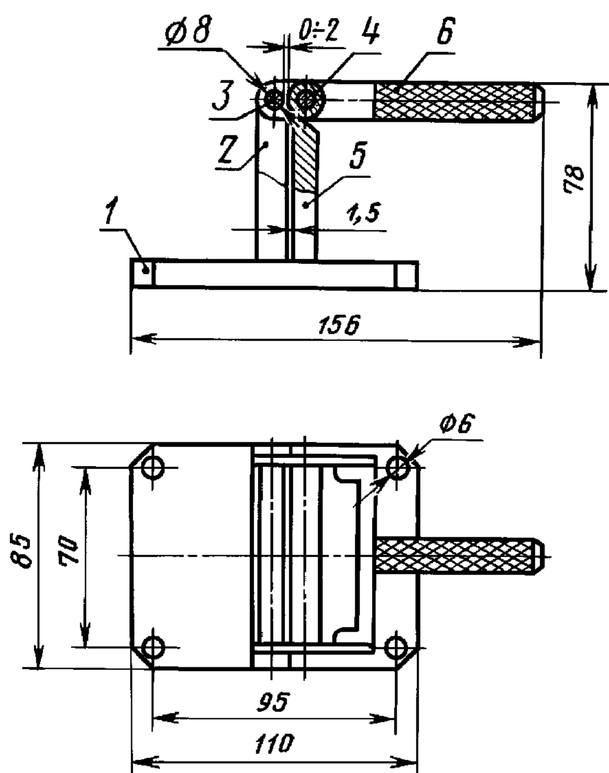
Приспособление для изгиба образцов
