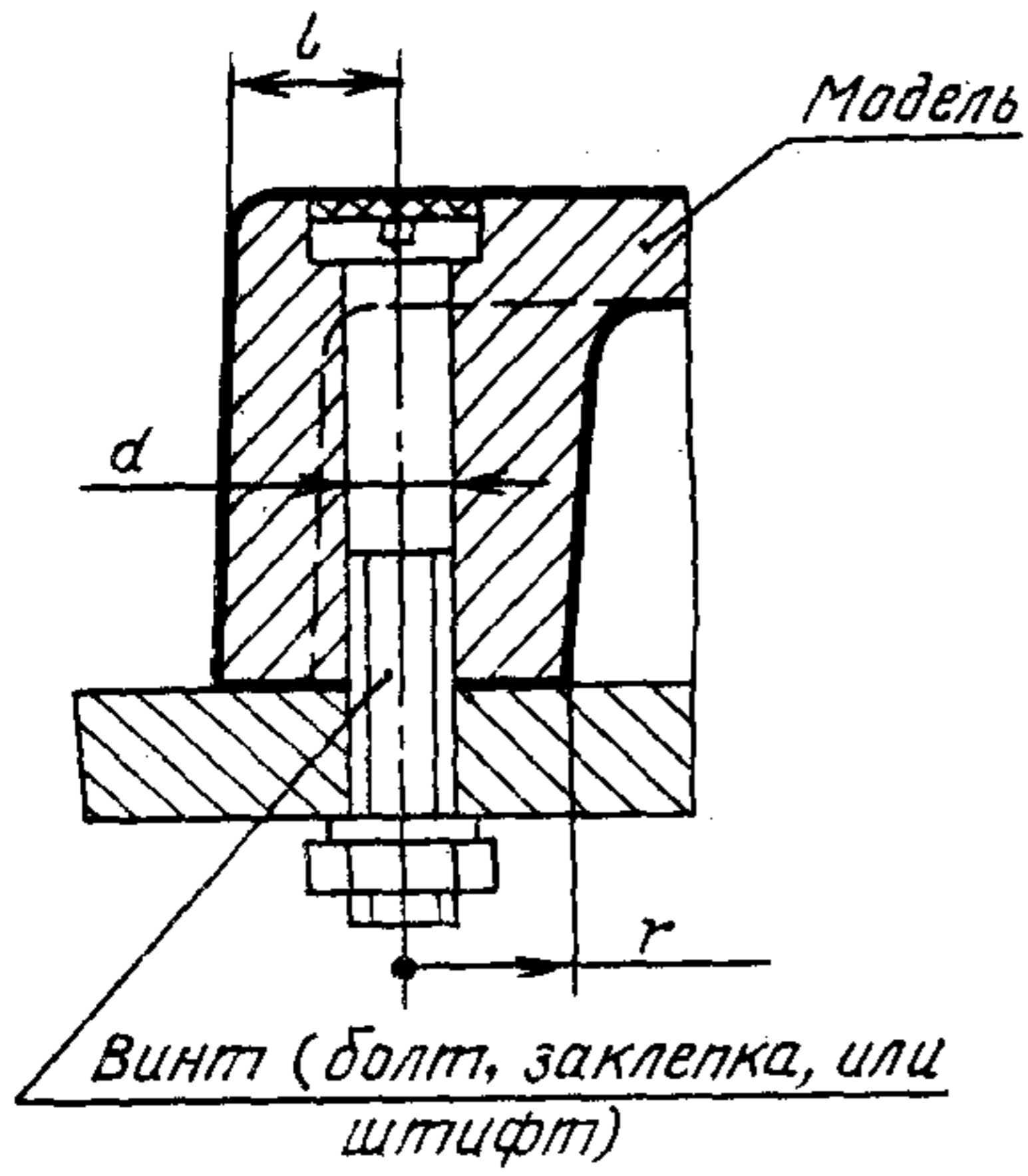
Исполнение 1
