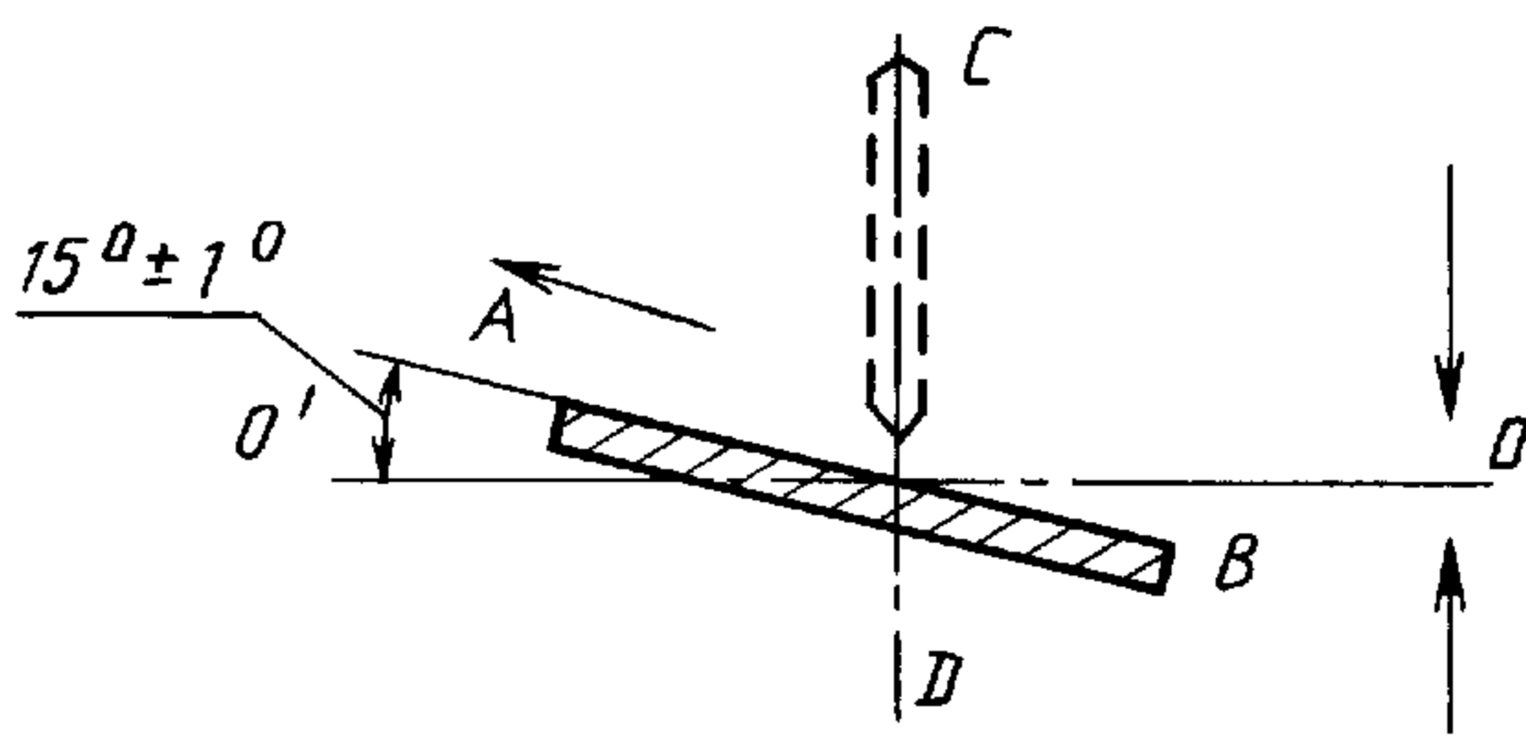
Взаимное расположение электродов
