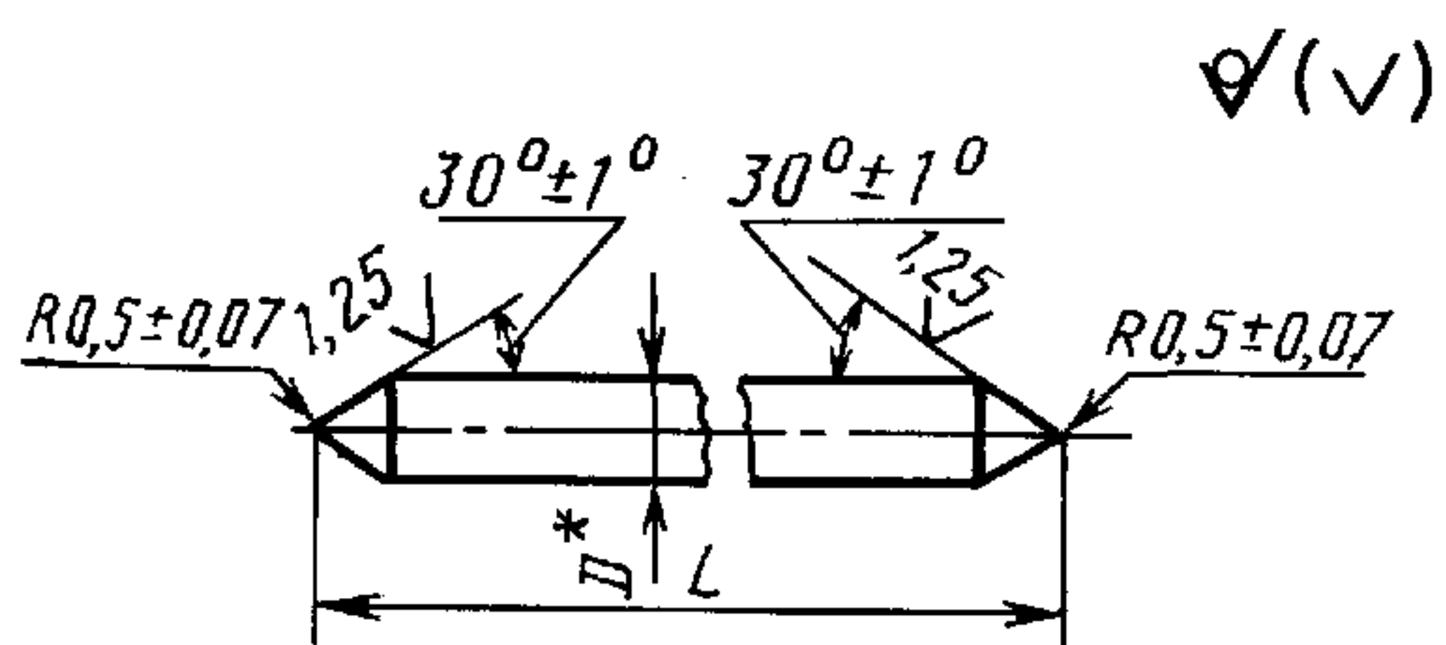
Стержень
