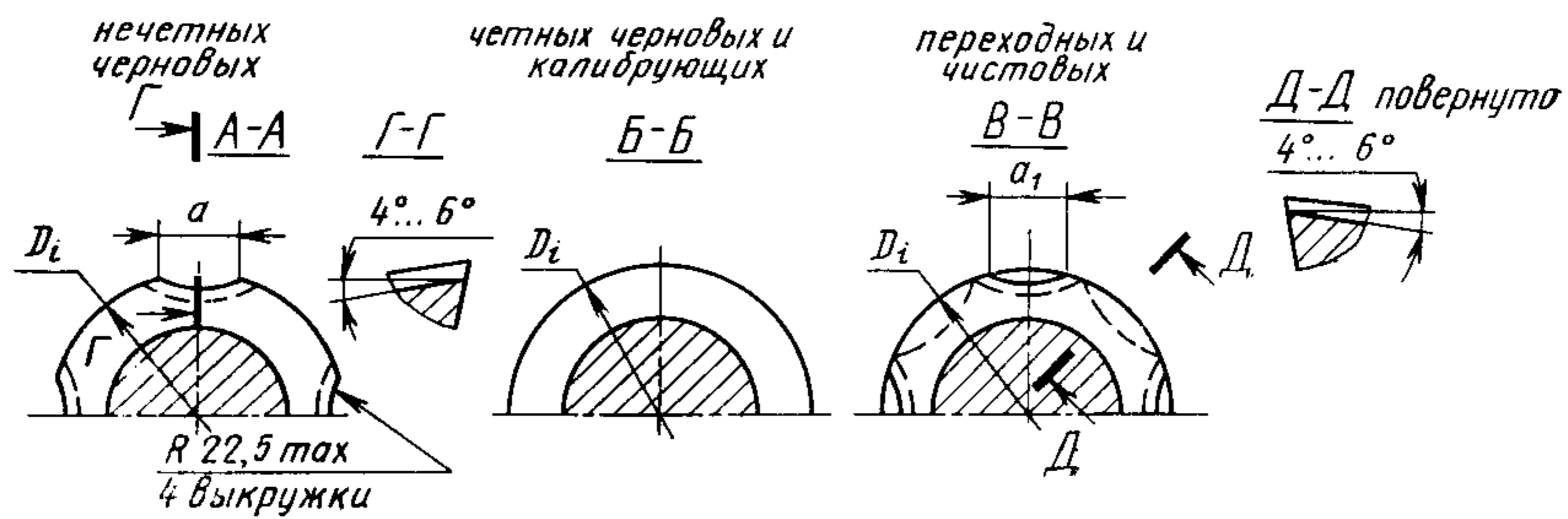
Форма зубьев и расположение выкружек на зубьях
