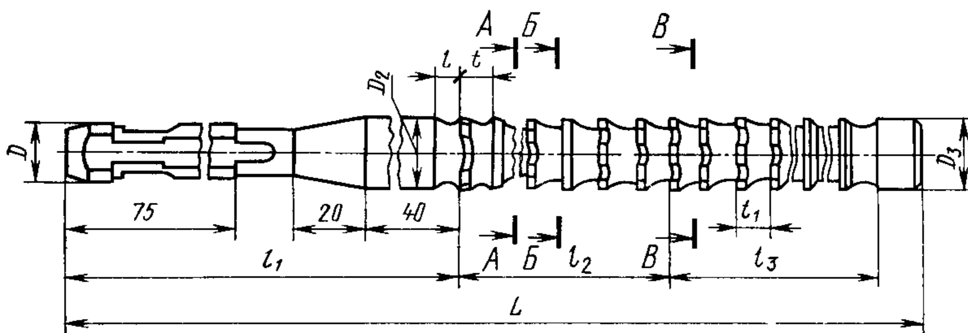
Форма зубьев и расположение выкружек на зубьях
