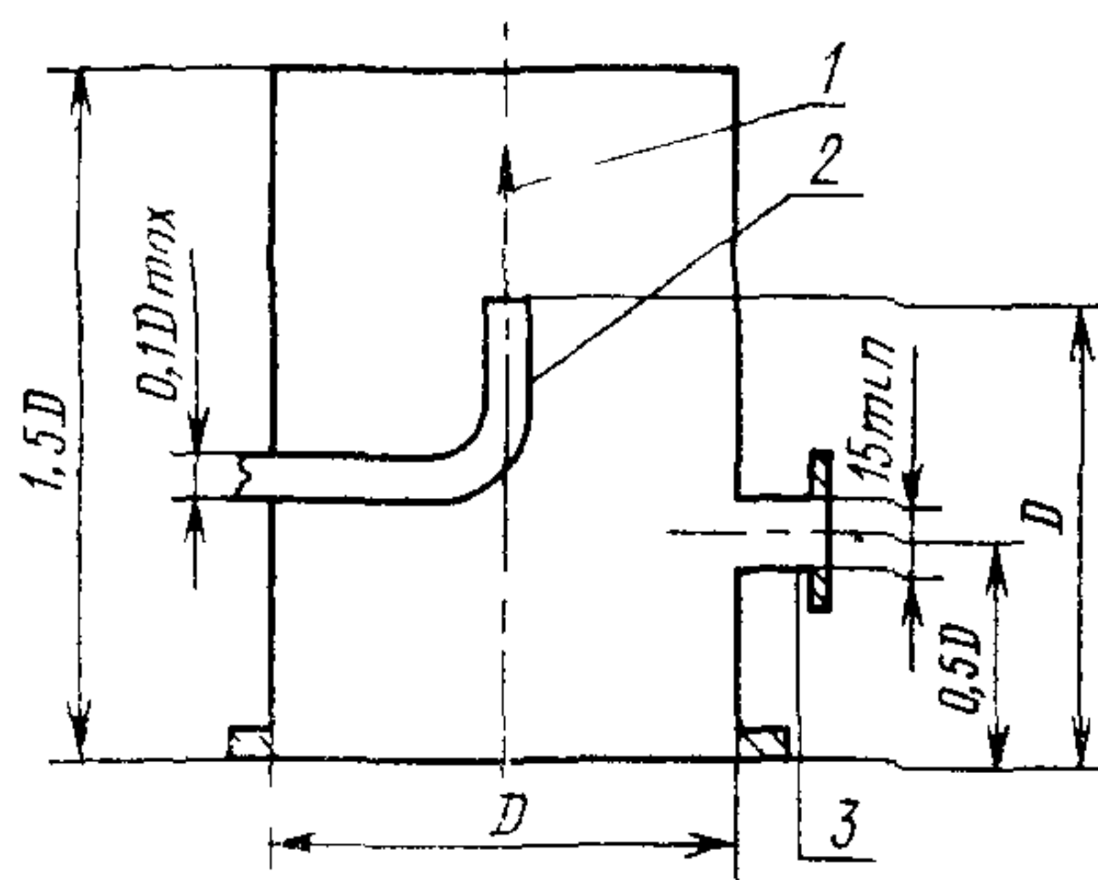
1—направление потока газа; 2—напускная трубка, 3—место подсоединения вакуумметра
