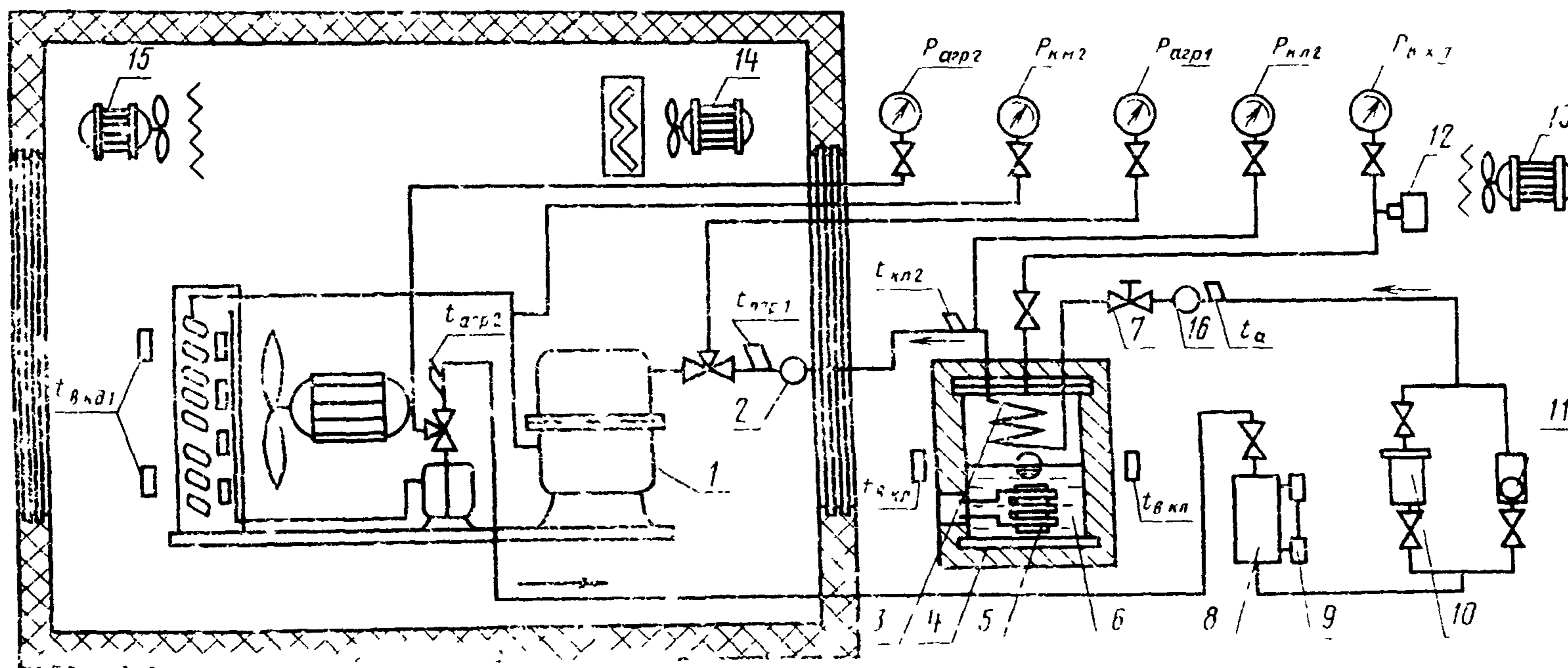
Схема стенда с электрическим калориметром
