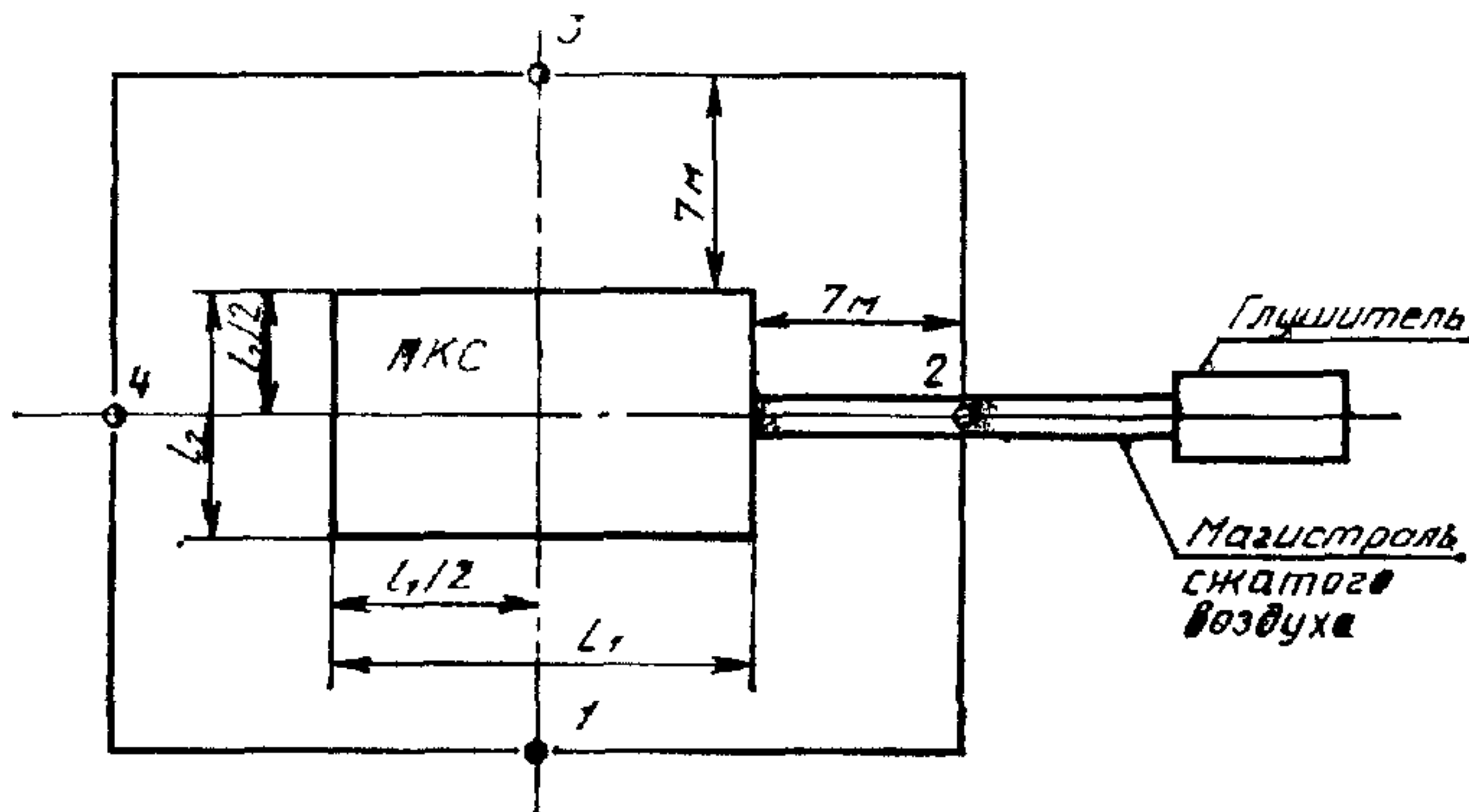
1—4 — точки измерения шума, l_1 и l_2 — длина и ширина сгибающего источника шума параллелепипеда
