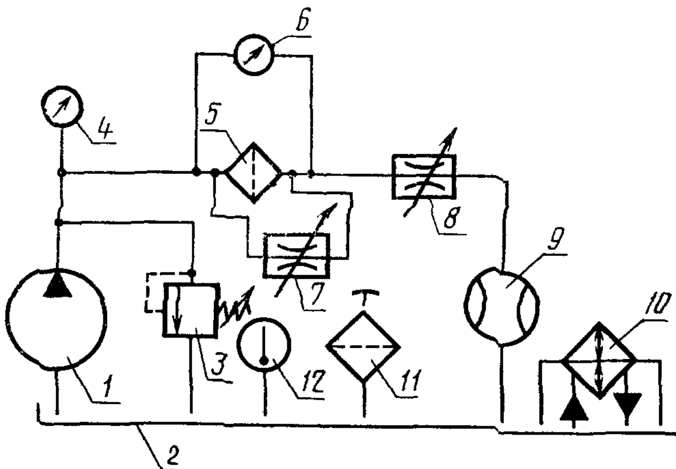
Схема стенда для проверки срабатывания индикатора загрязненности
