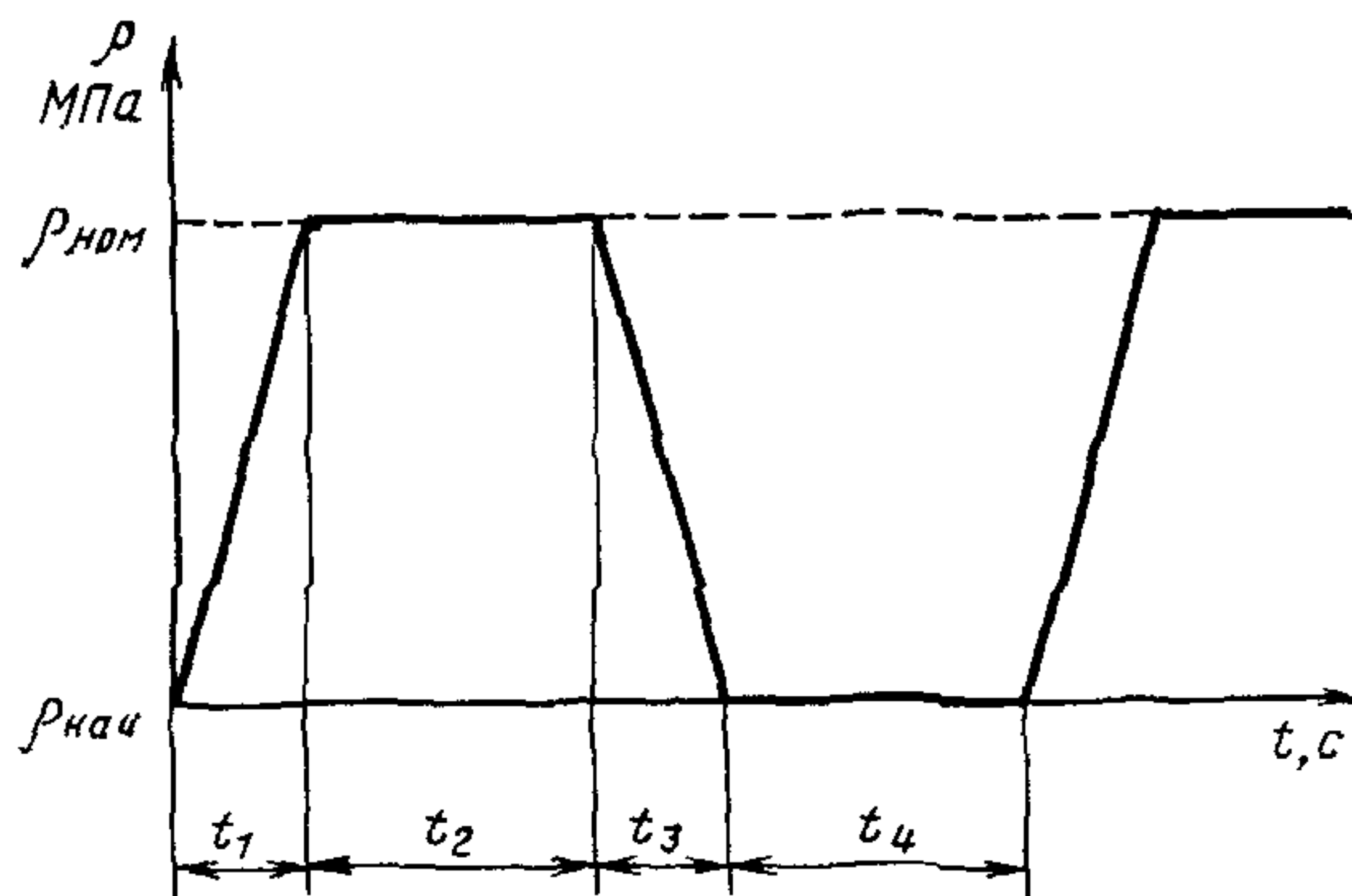
Циклограмма нагружения корпуса фильтра при ресурсных испытаниях
