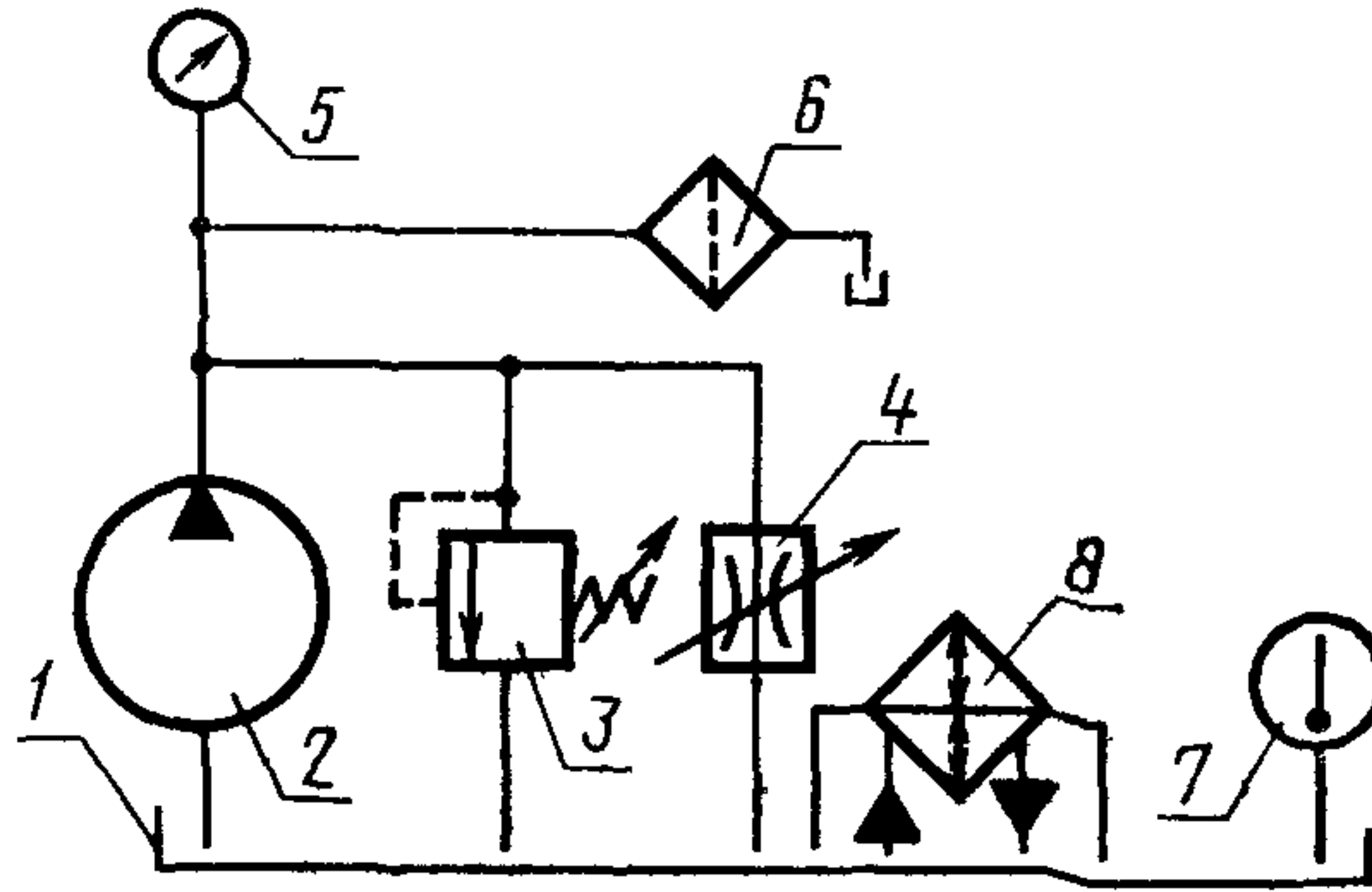
Схема стенда для проверки срабатывания предохранительного клапана
