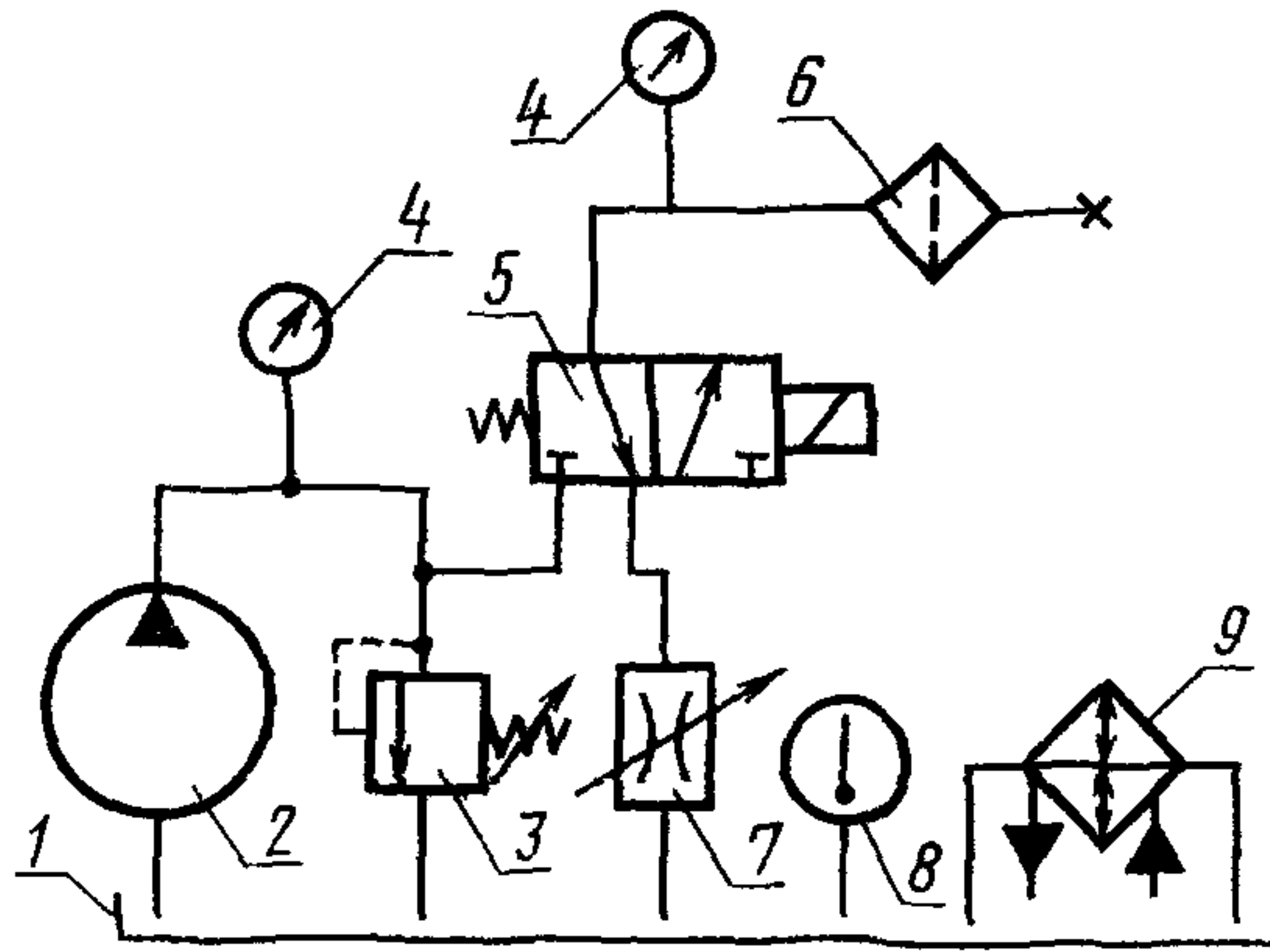
Схема стенда для ресурсных испытаний фильтра
