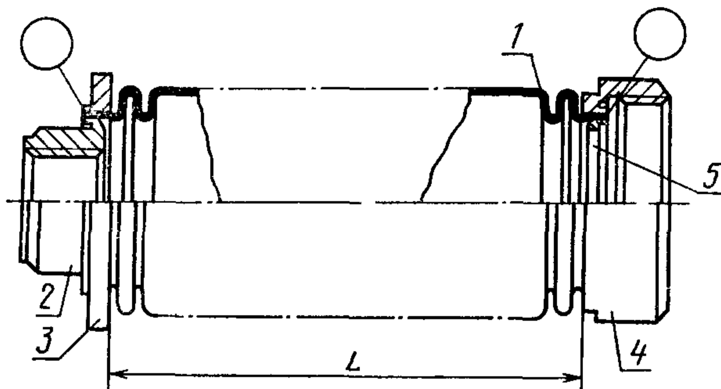
1—сильфон; 2—втулка; 3—кольцо; 4—втулка, 5—кольцо
