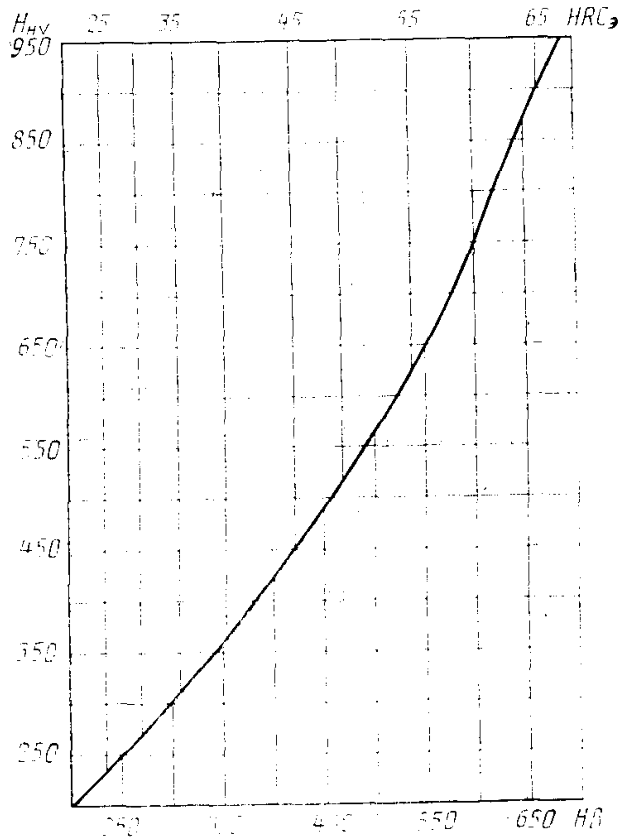
График соотношений твердостей, выраженных в единицах HB, HRC 3 и HV
