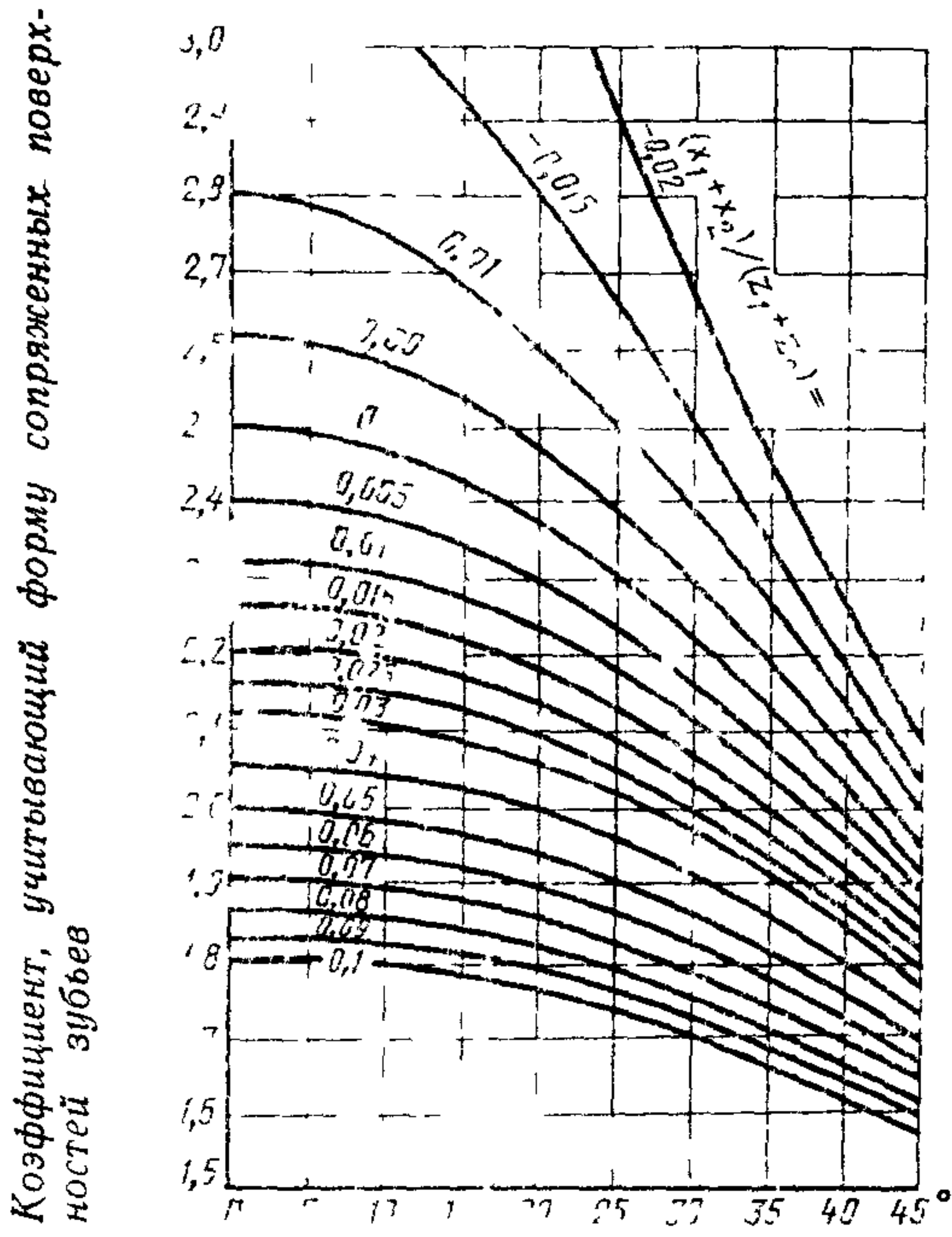
Угол наклона на делительном цилиндре
