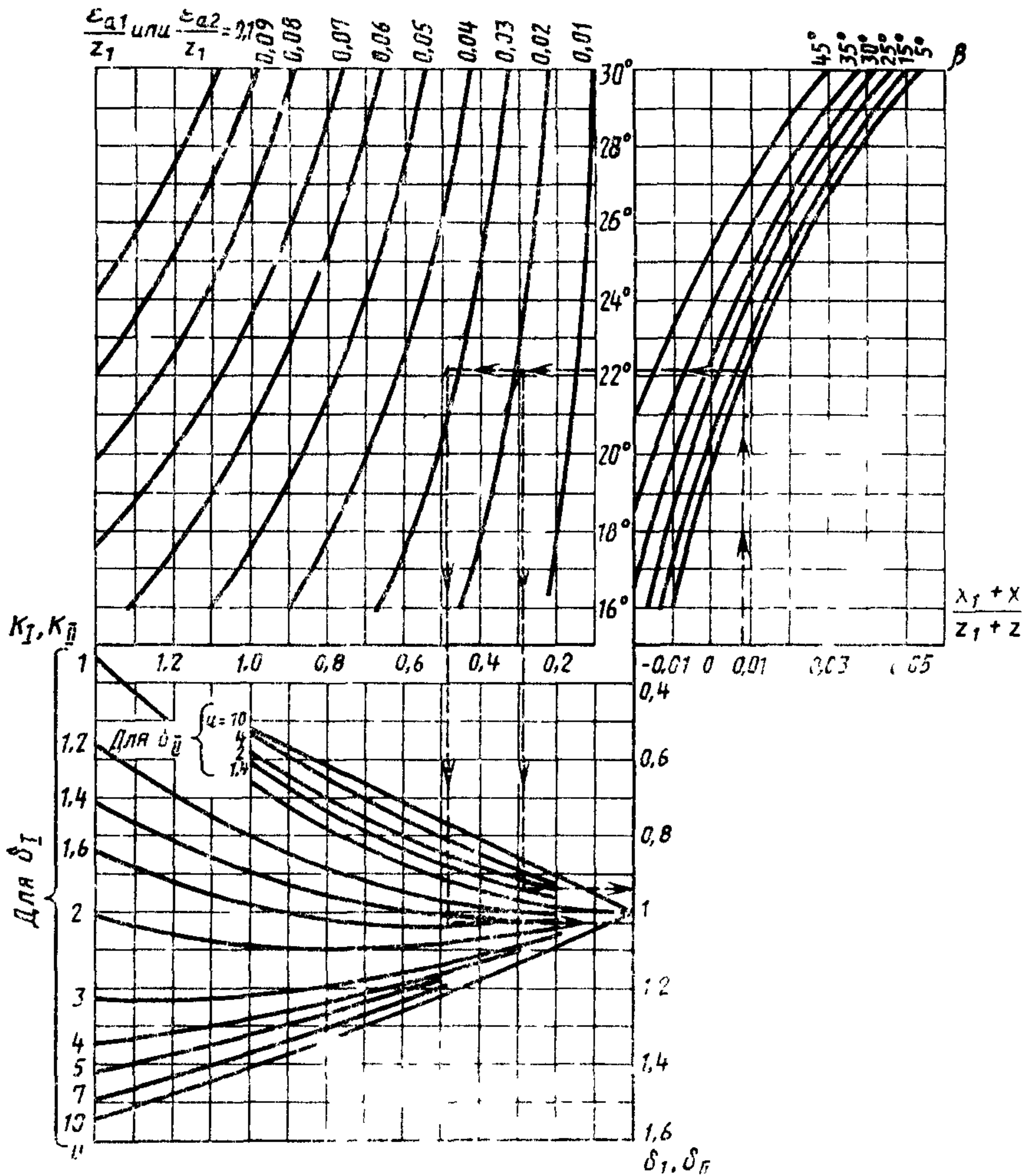
График для определения коэффициентов \delta_I и \delta_{II}
