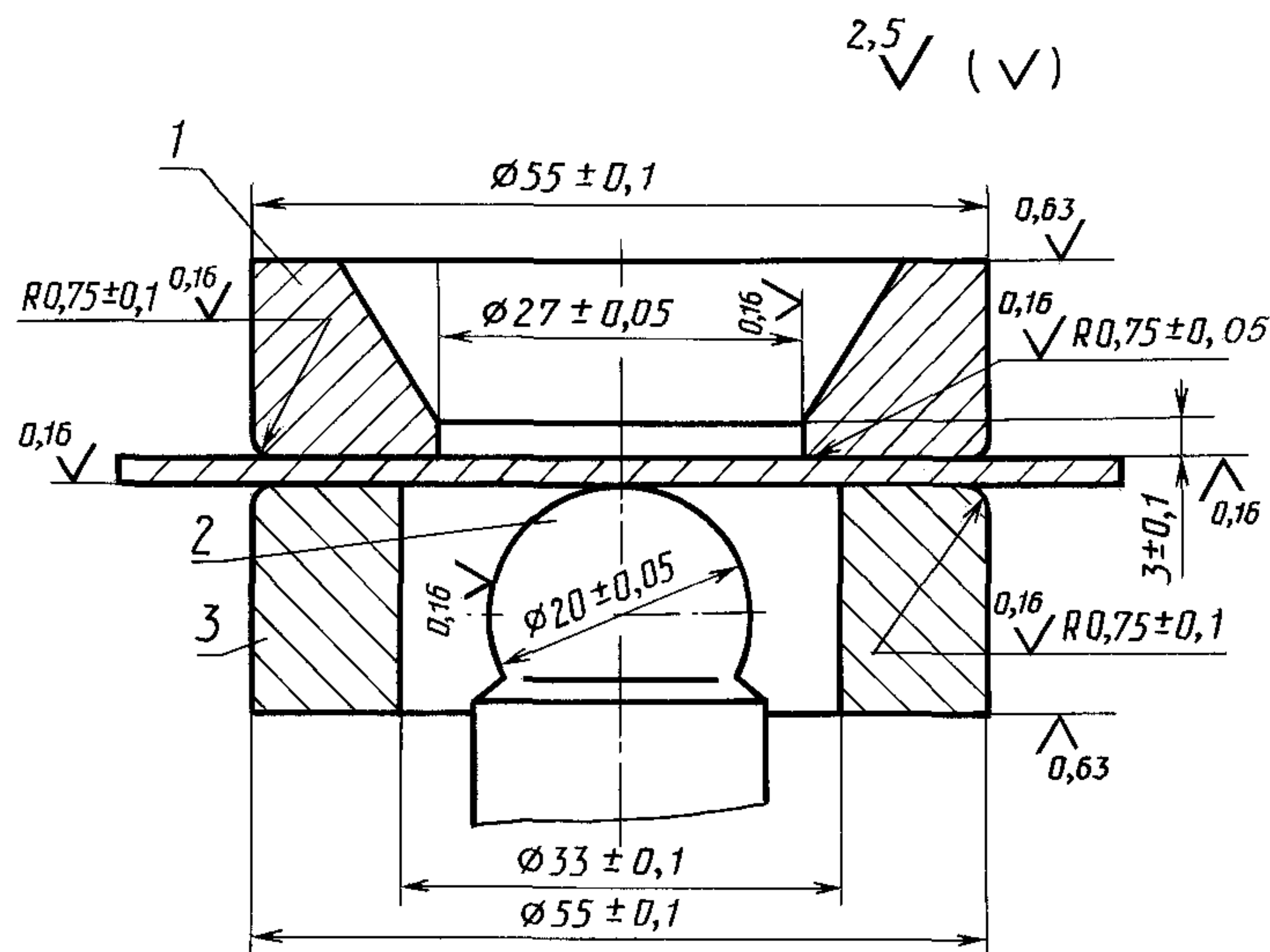
1 — матрица; 2 — пуансон; 3 — прижимное кольцо
