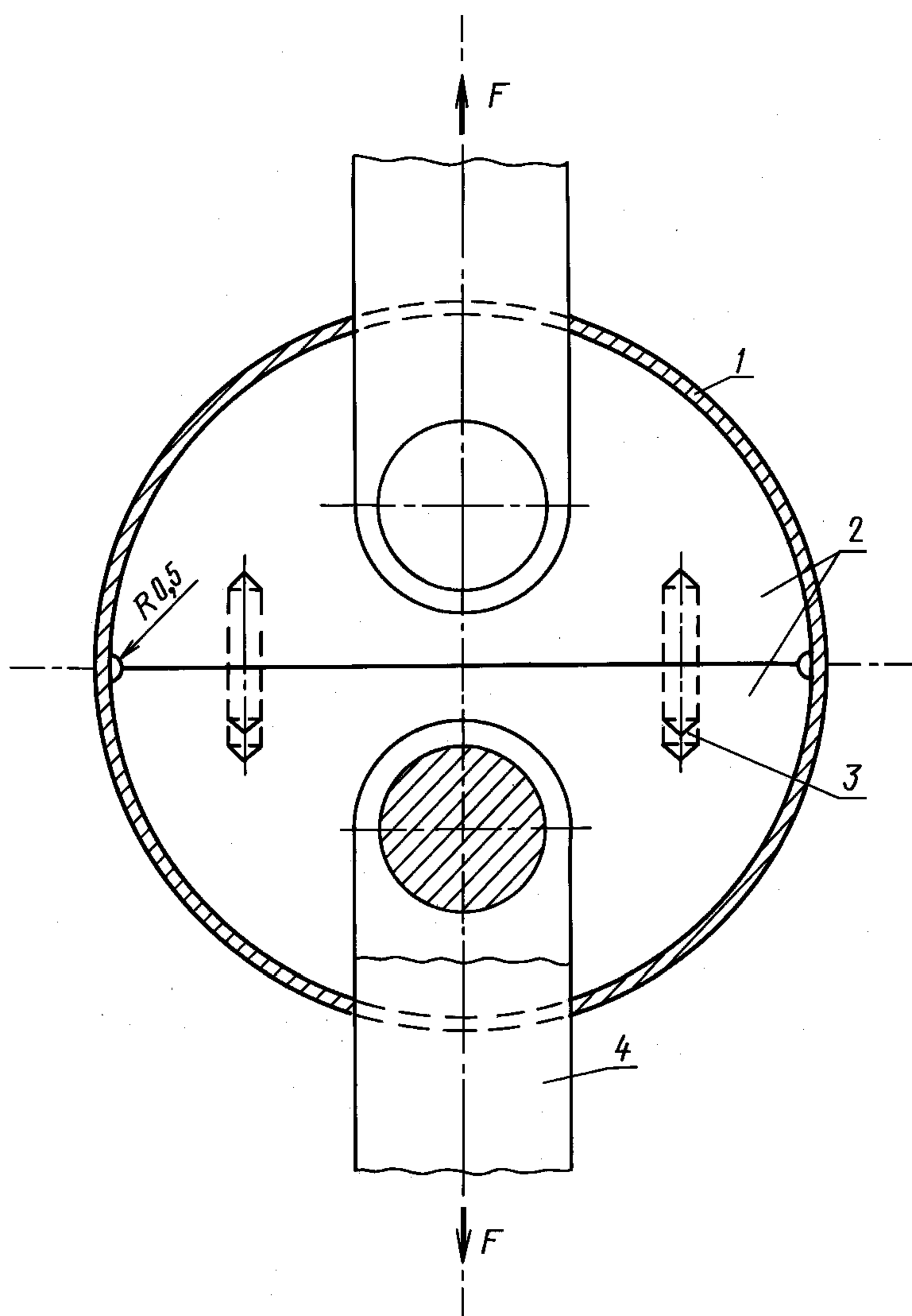
1 — образец; 2 — полудиски; 3 — направляющая; 4 — тяга
