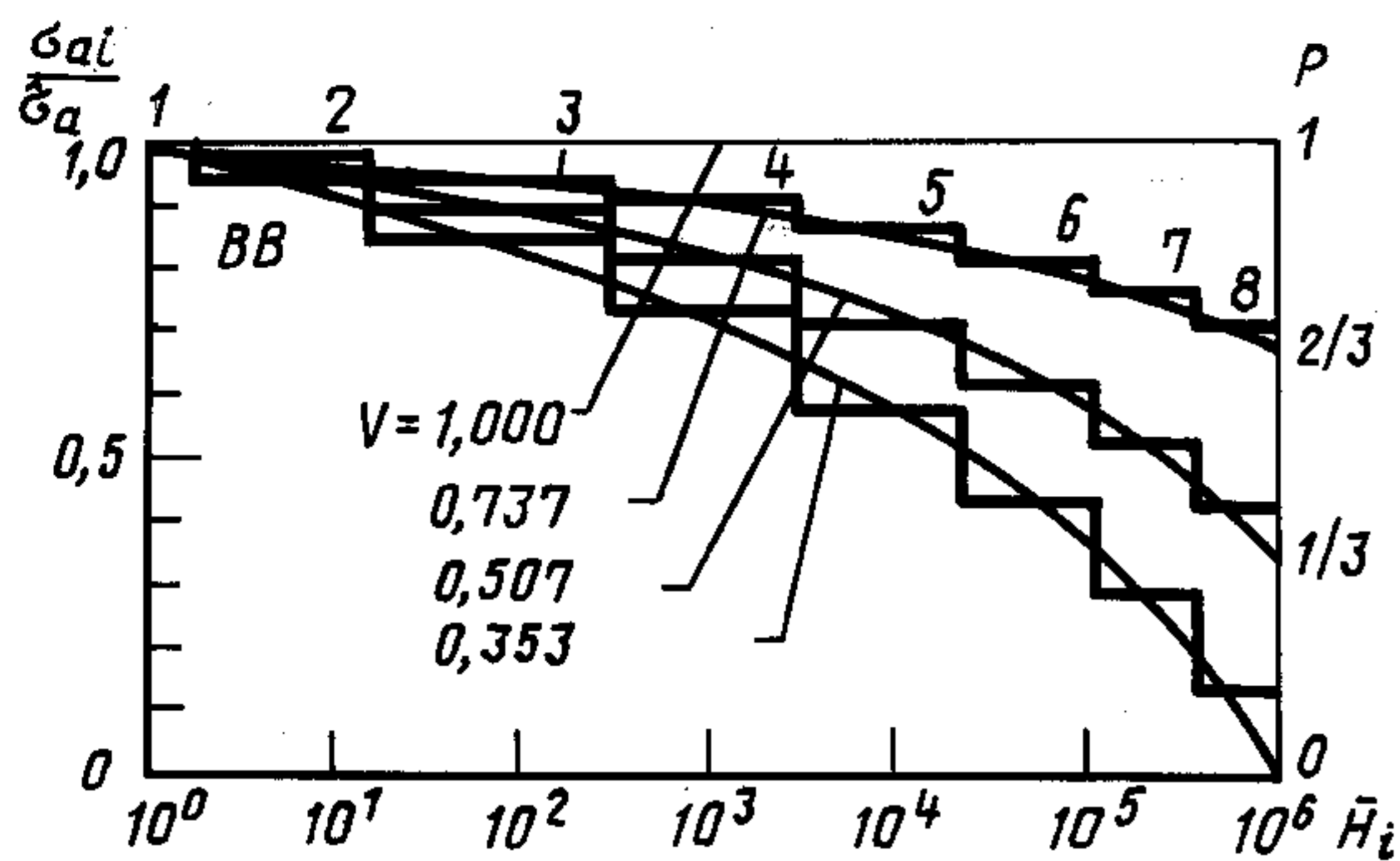
Биномиальное распределение (BB)
