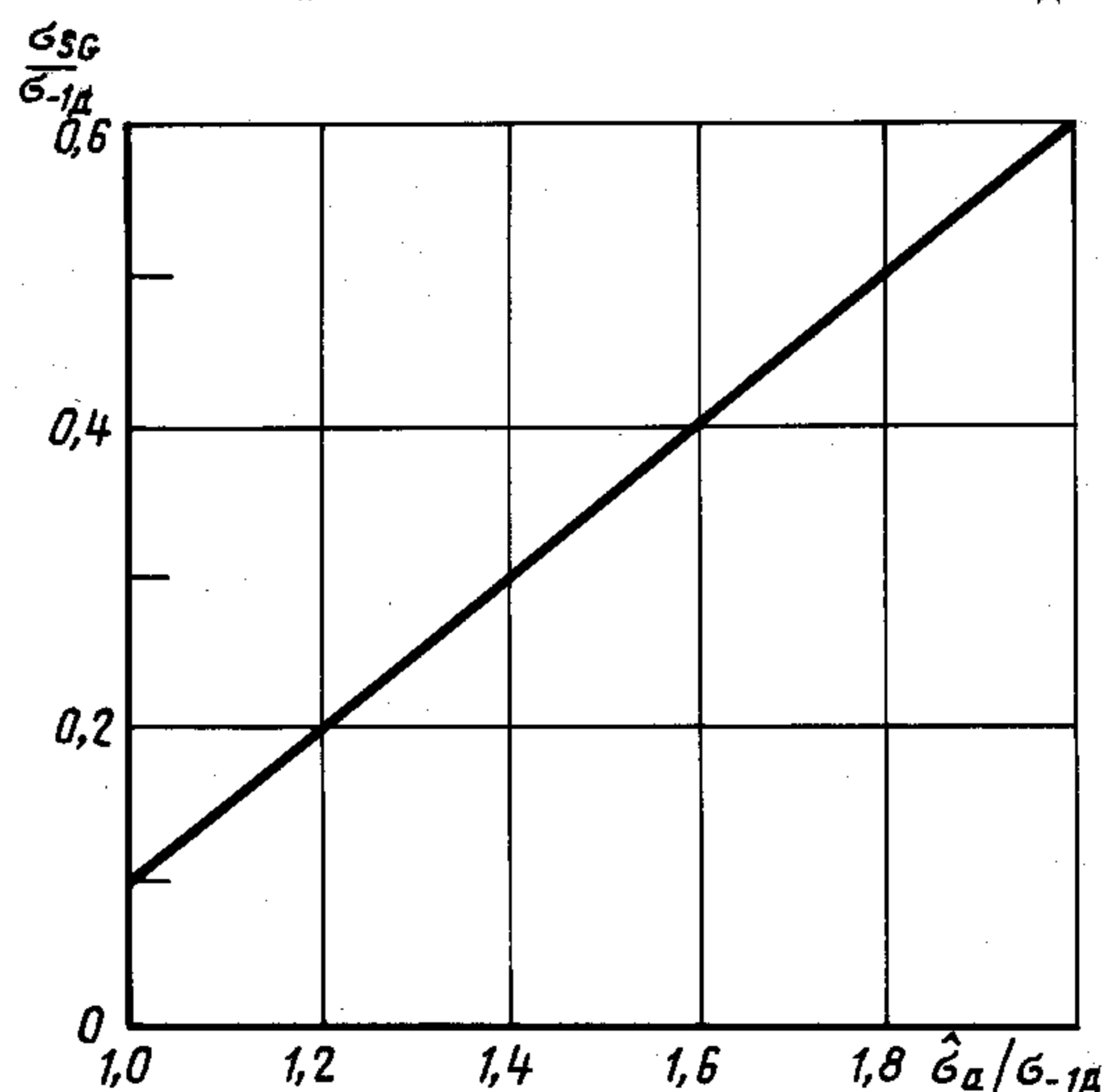
Значения повреждающих амплитуд \sigma_{SG} в зависимости от максимальной амплитуды спектра \hat{\sigma}_a и предела выносливости \sigma_{-1д}
