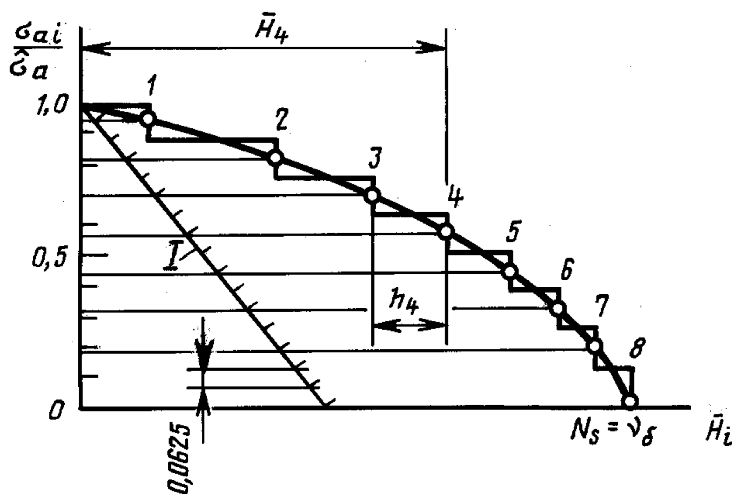
Линейное разбиение спектра нагружения на 8 ступеней
