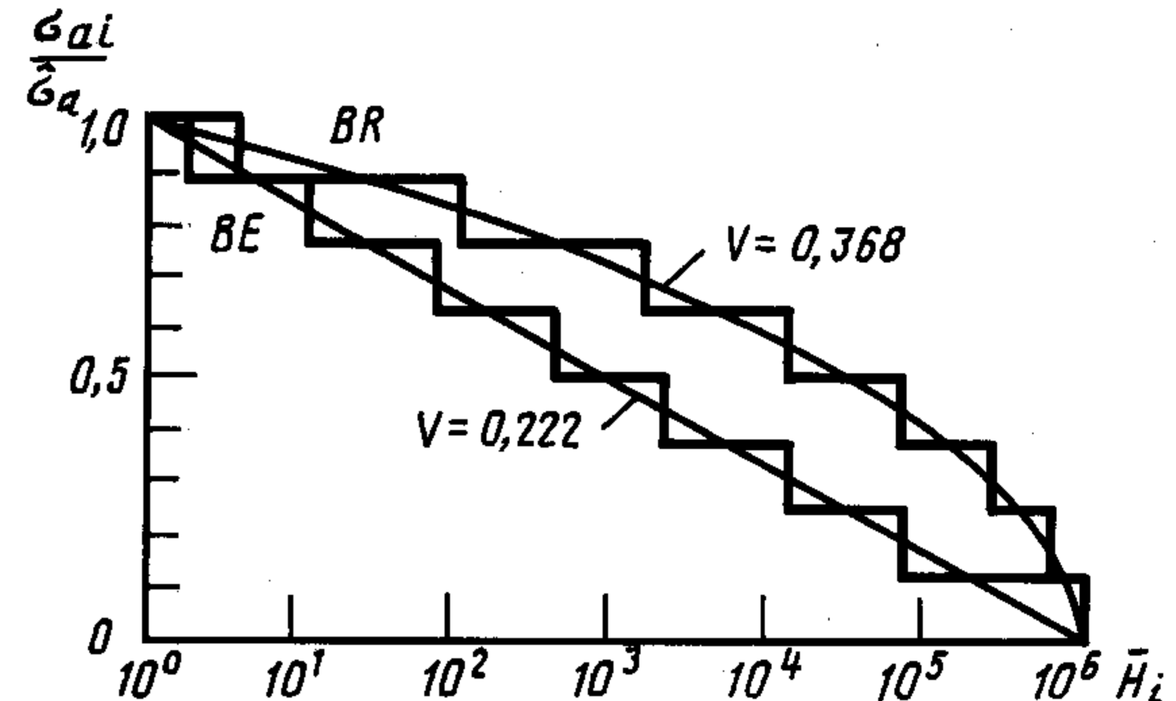
Распределения Рэлея (BR) и экспоненциальное (BE)
