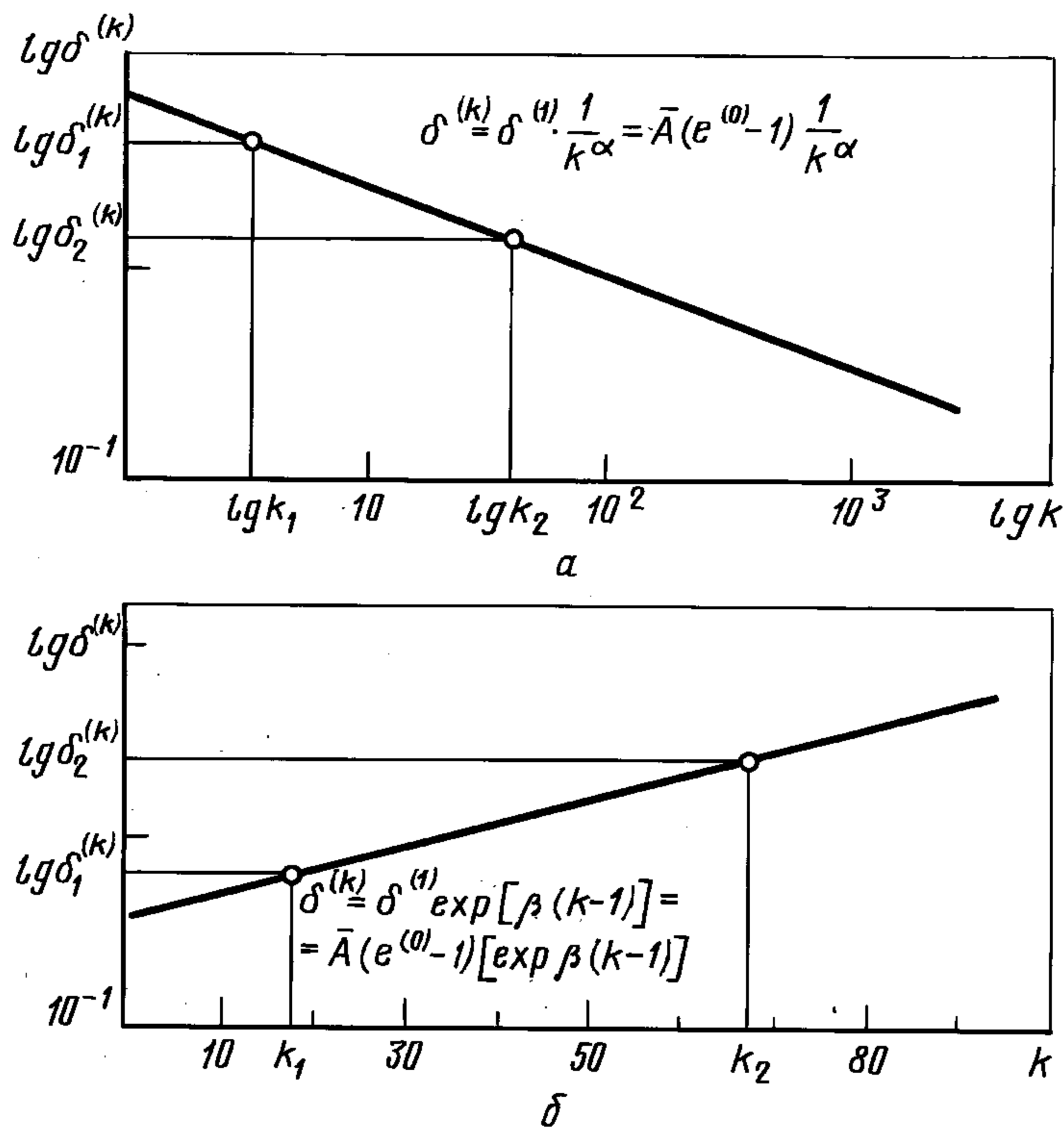
а — циклическое упрочнение; б — циклическое разупрочнение
