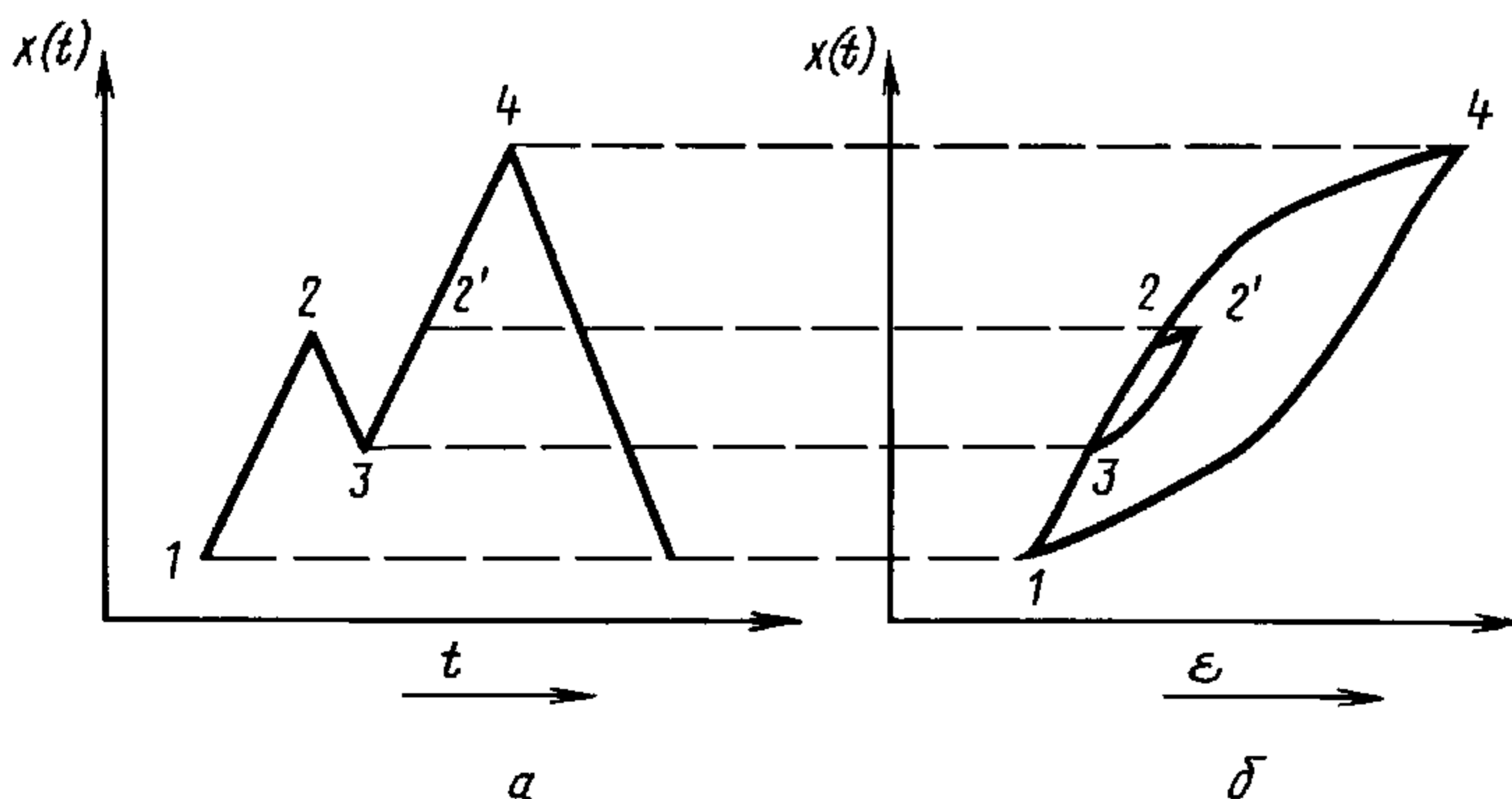
a — фрагмент процесса нагружения; б — диаграмма «напряжение—деформация»
