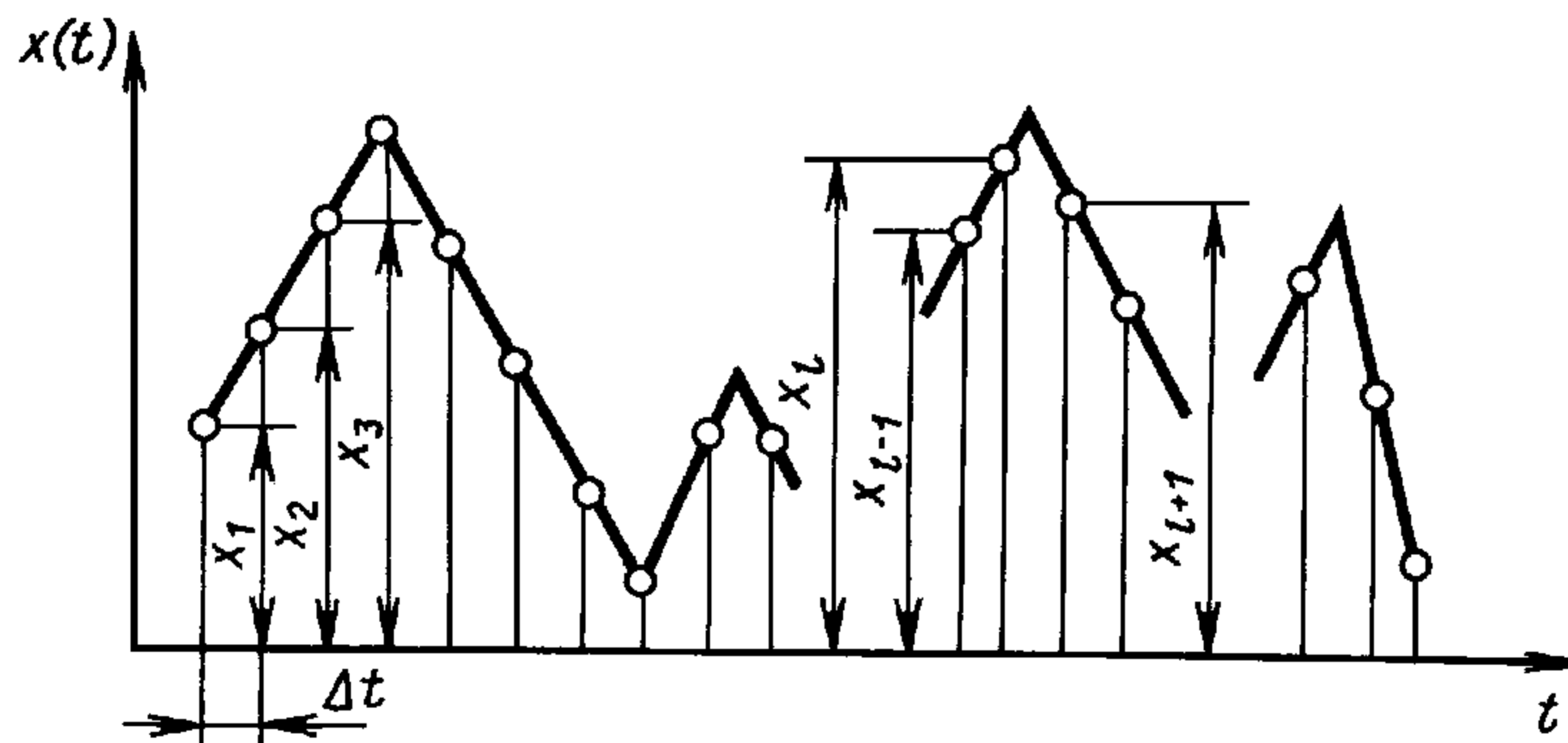
Дискретизация по методу случайных ординат
