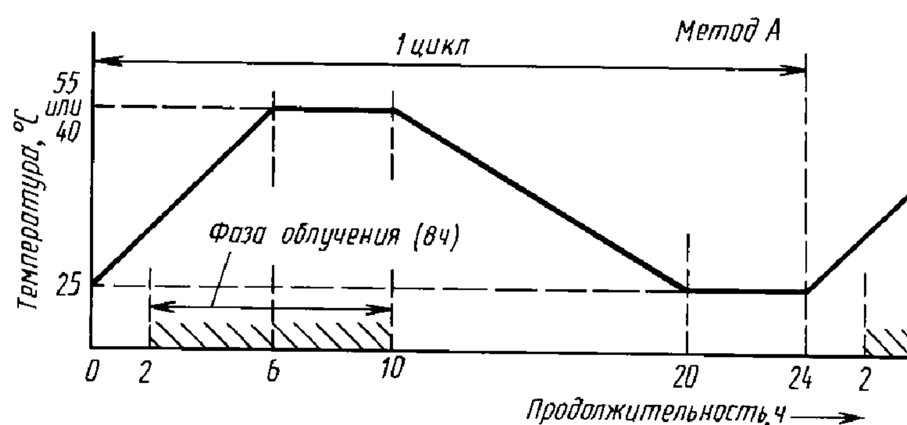
Режим облучения и зависимость температуры от времени
