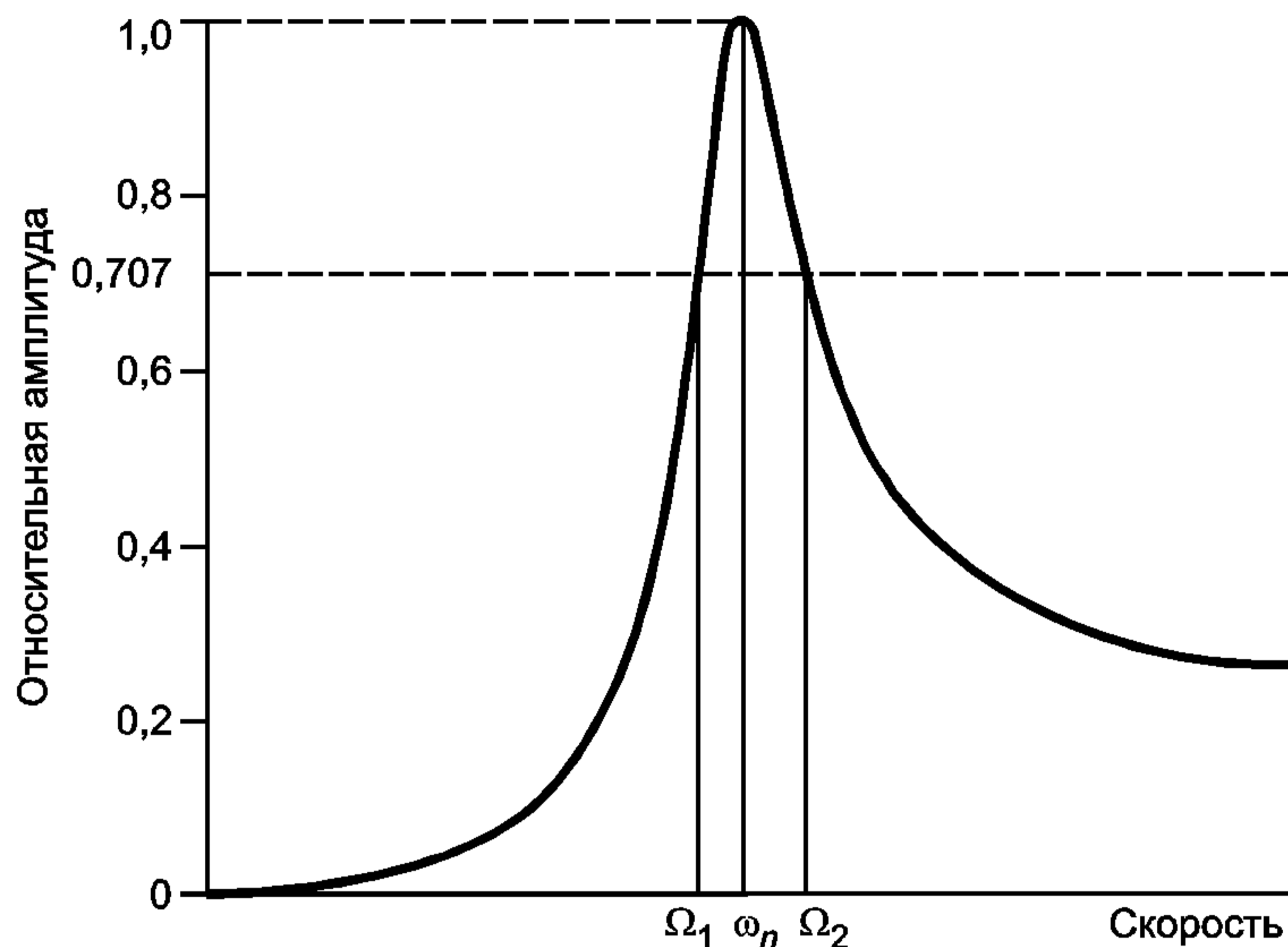
Рисунок 5 — Диаграмма Бодэ для оценки модальной чувствительности
