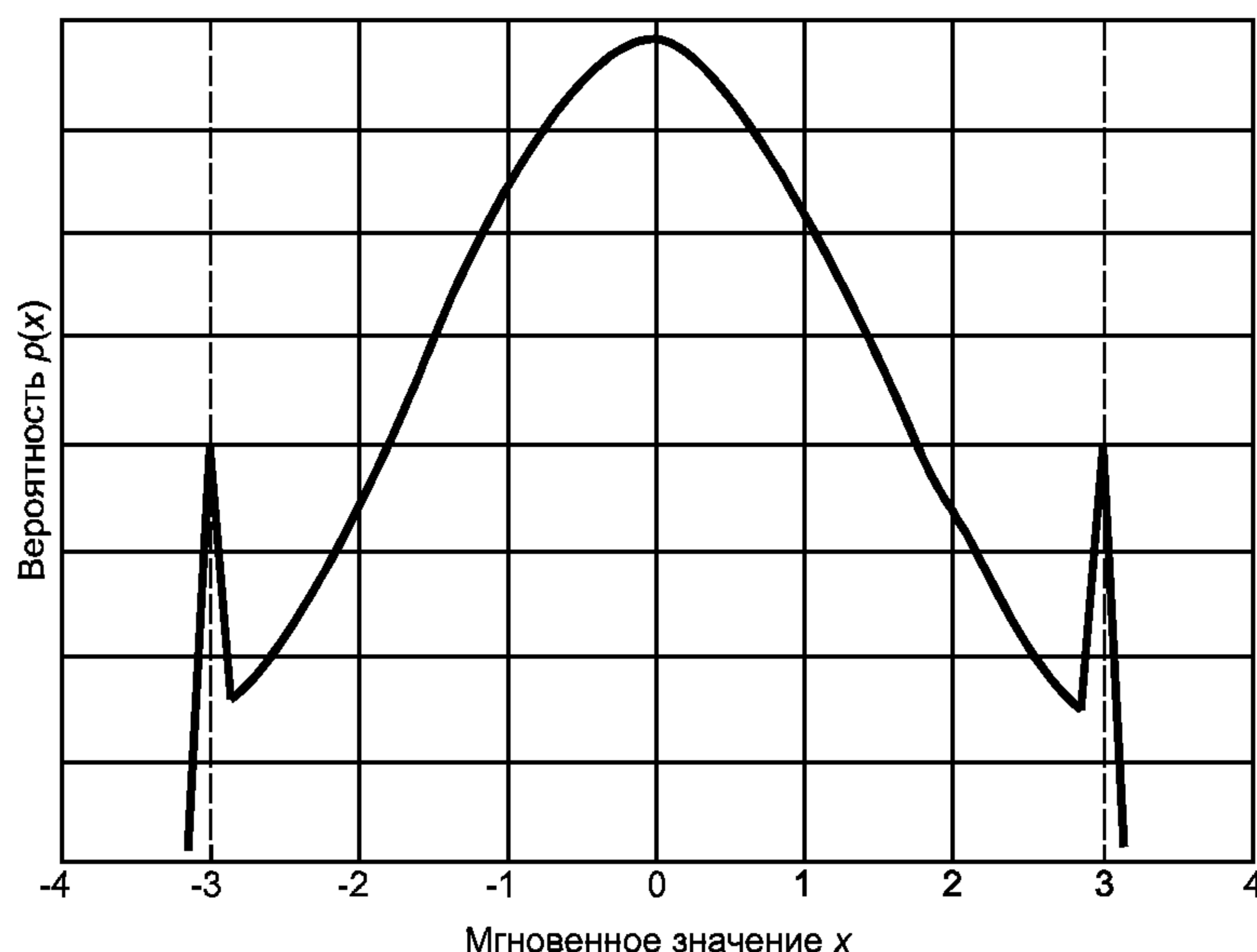
Рисунок А.3 — Негассовская плотность вероятности распределения
