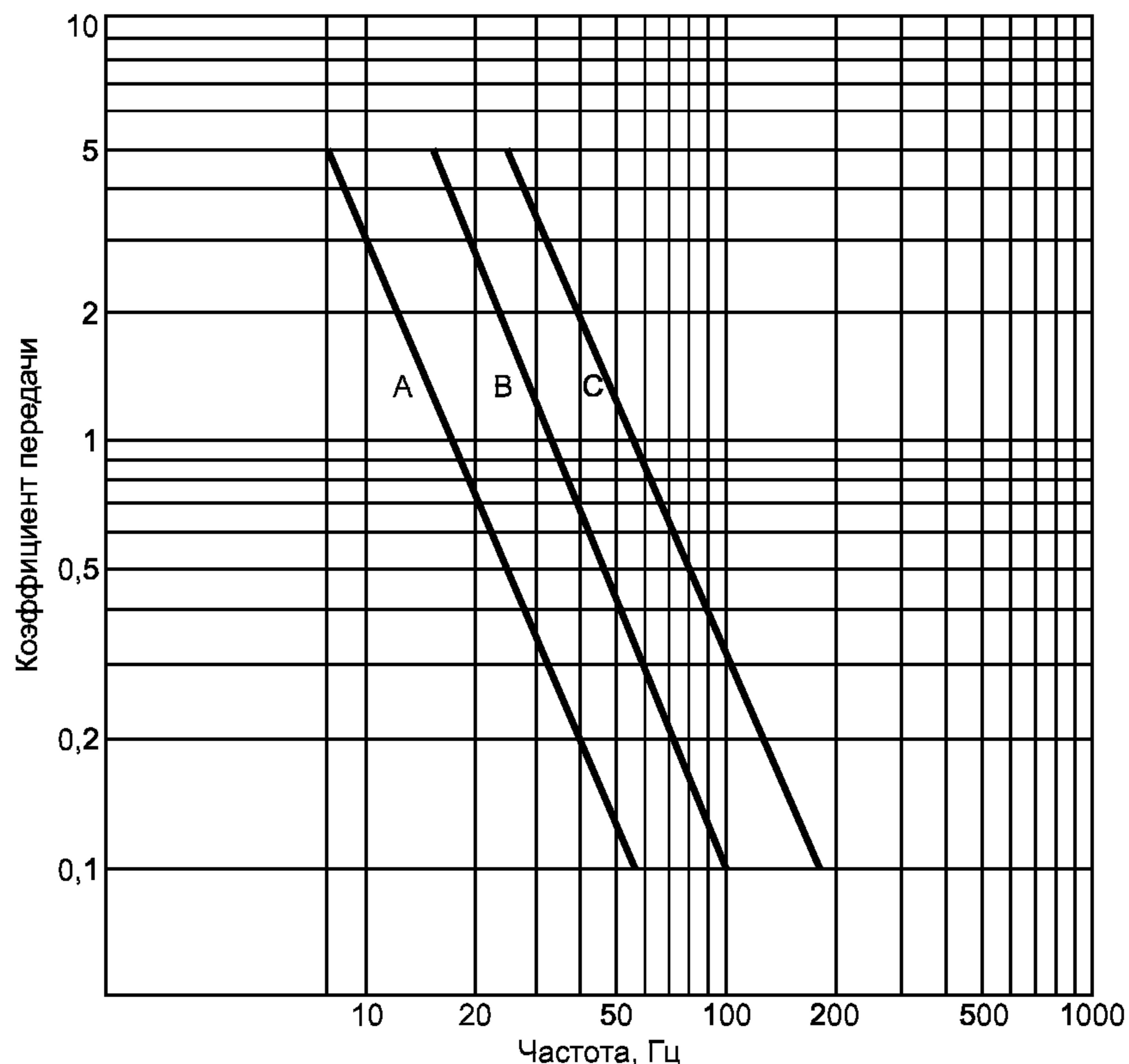
Рисунок А.6 — Коэффициент передачи виброизолятора
