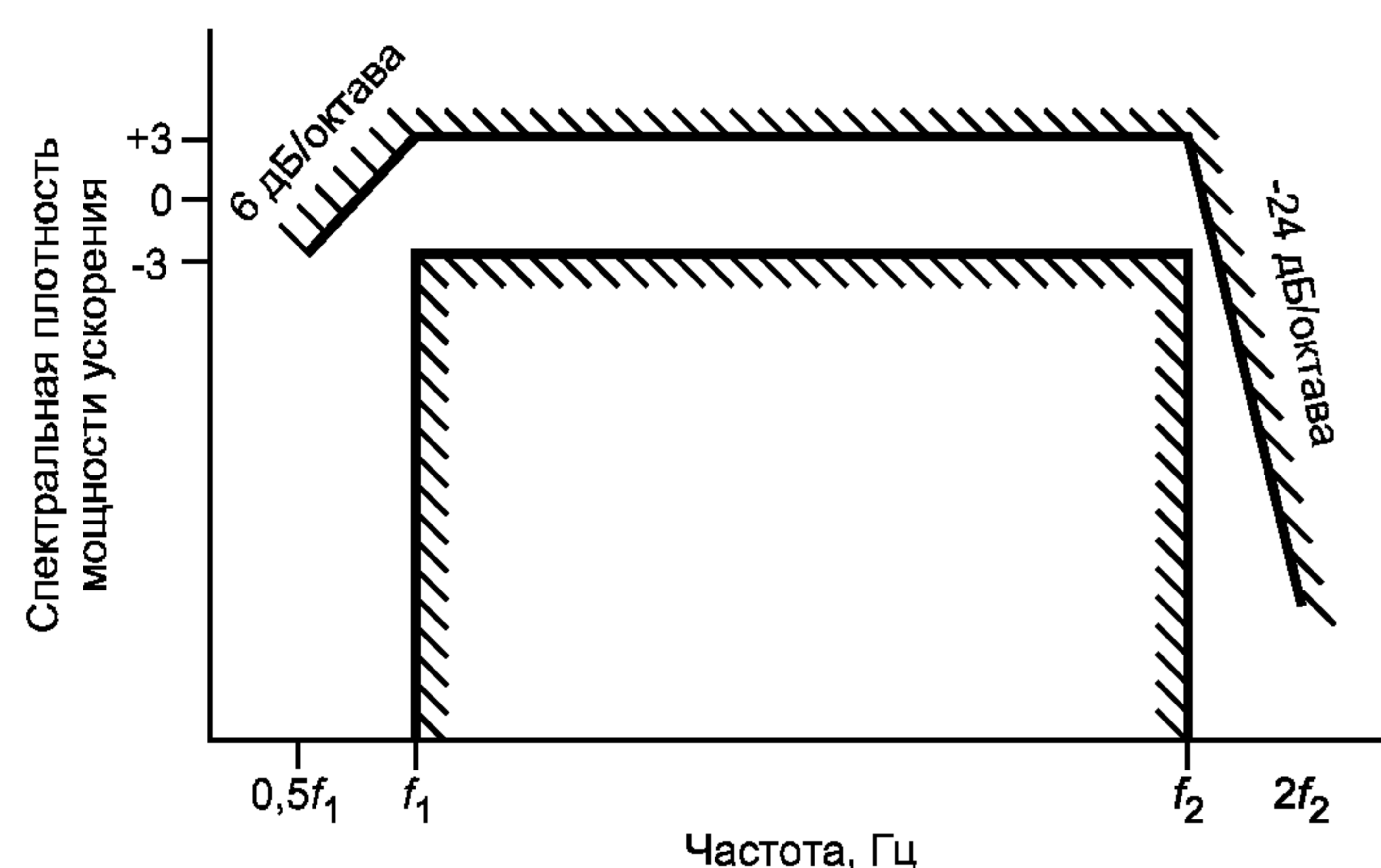
Рисунок 2 — Границы допуска для спектральной плотности мощности ускорения
