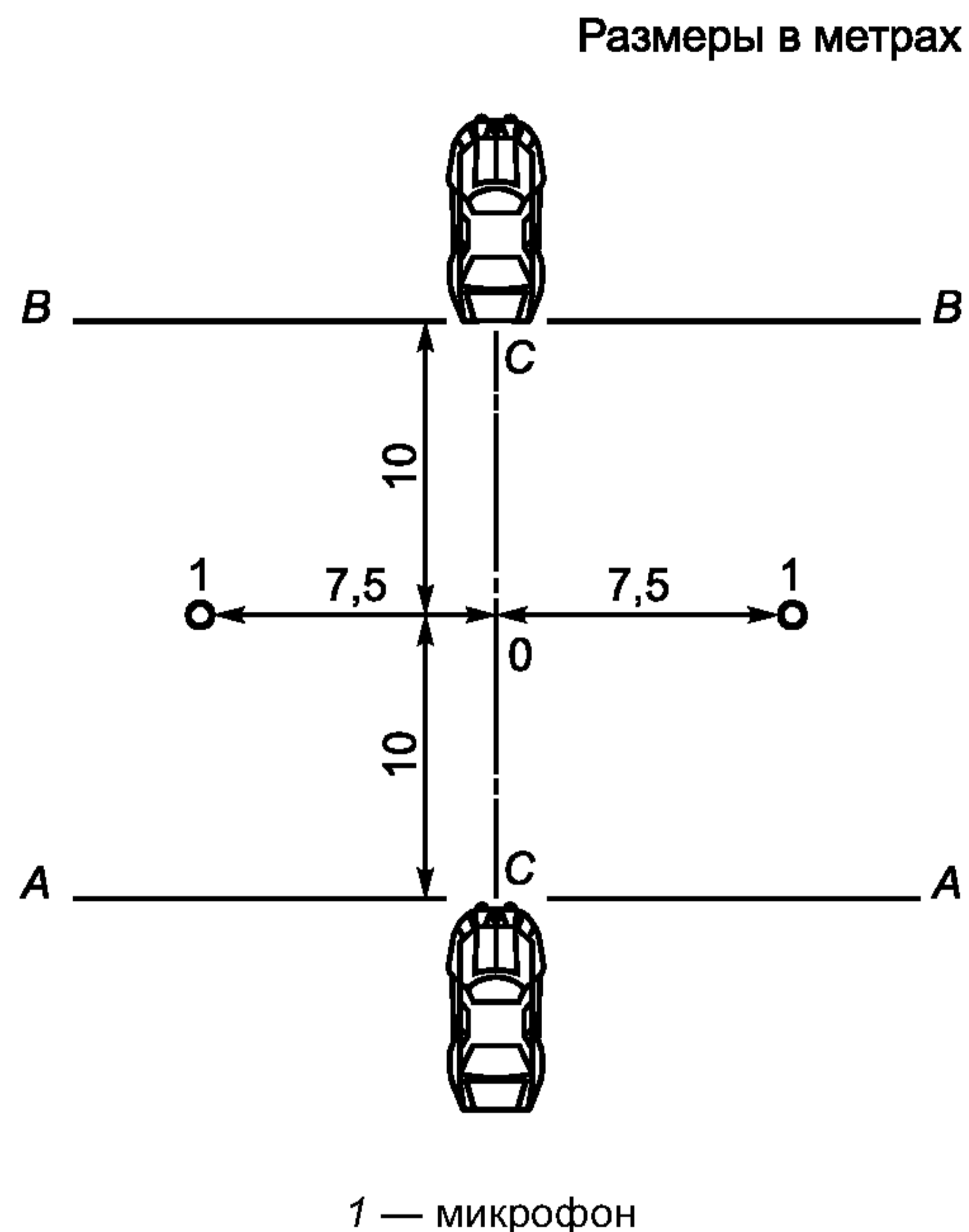
Рисунок 2 — Местоположения микрофонов
