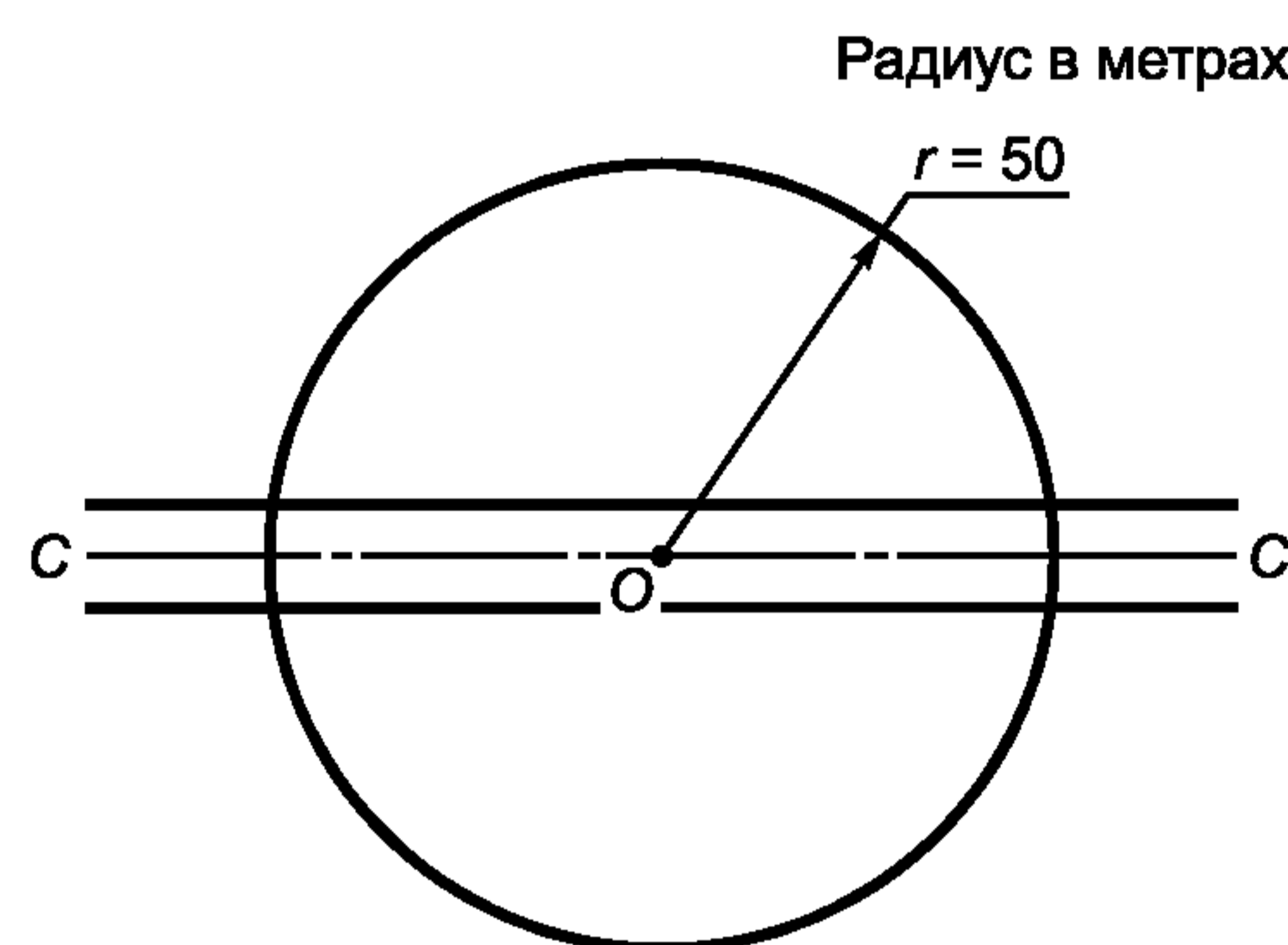
Рисунок 1 — Место испытаний
