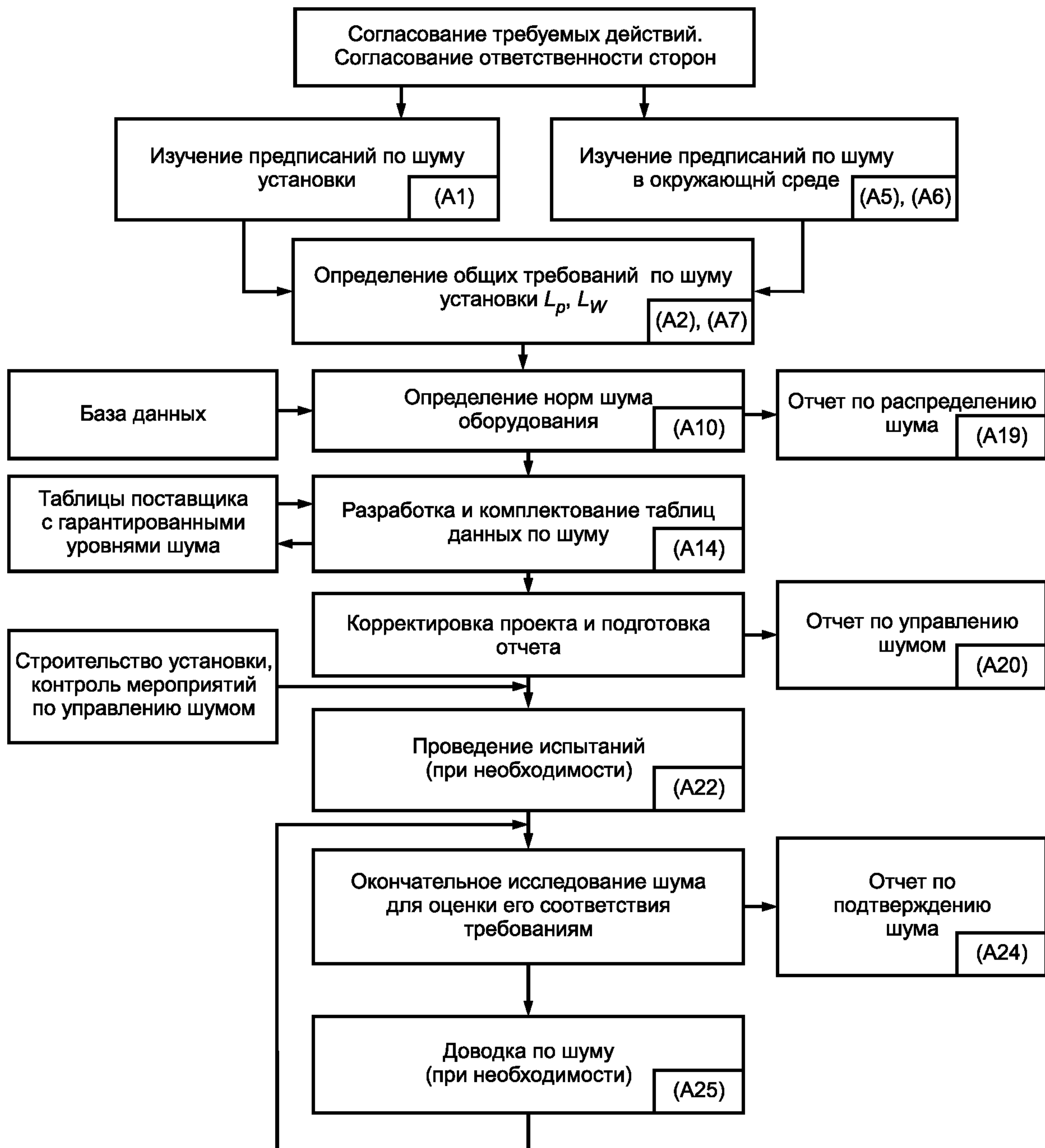
Рисунок А.1 — Схема управления шумом
