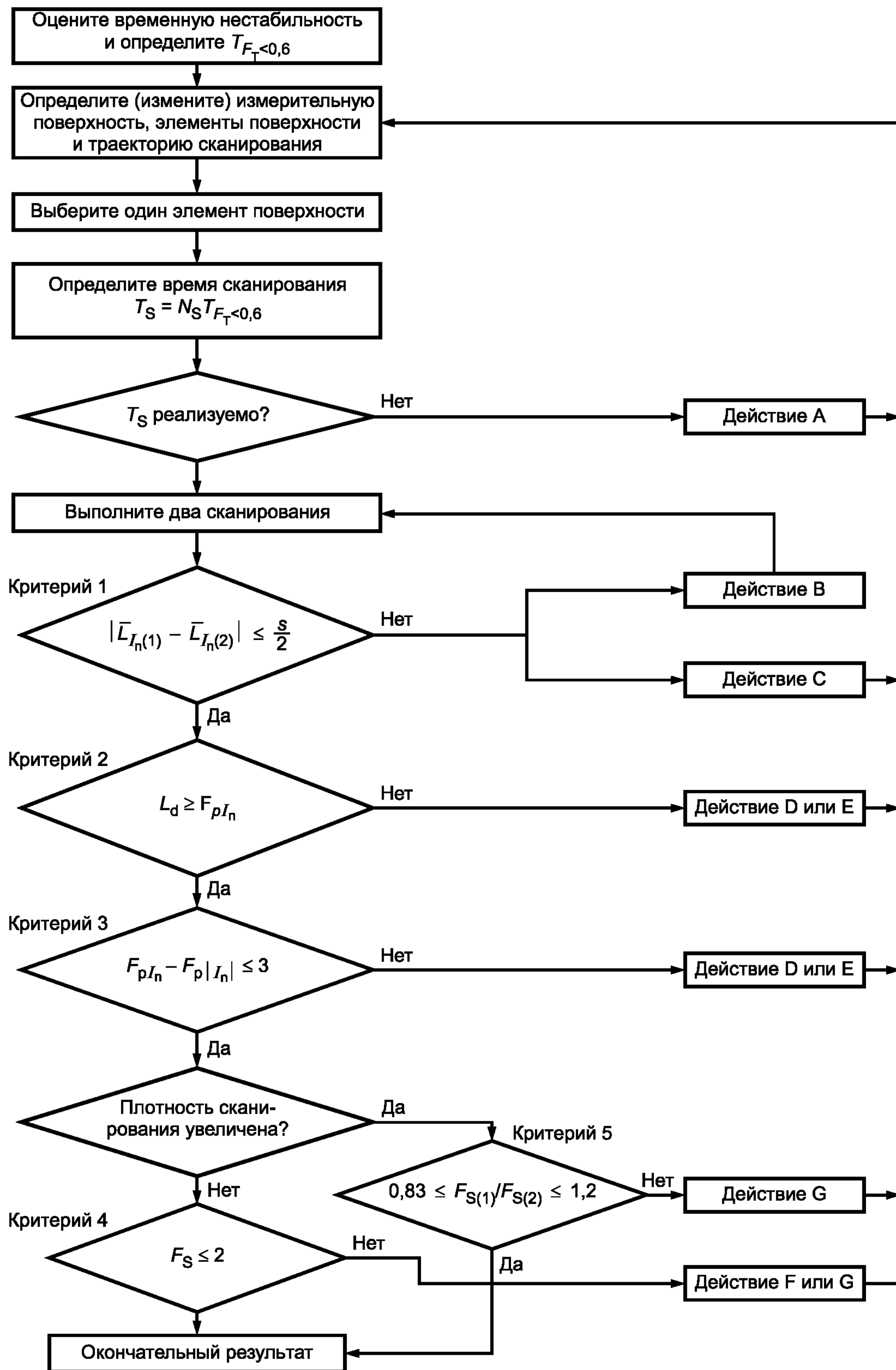
Рисунок С.1 — Алгоритм достижения необходимой точности
