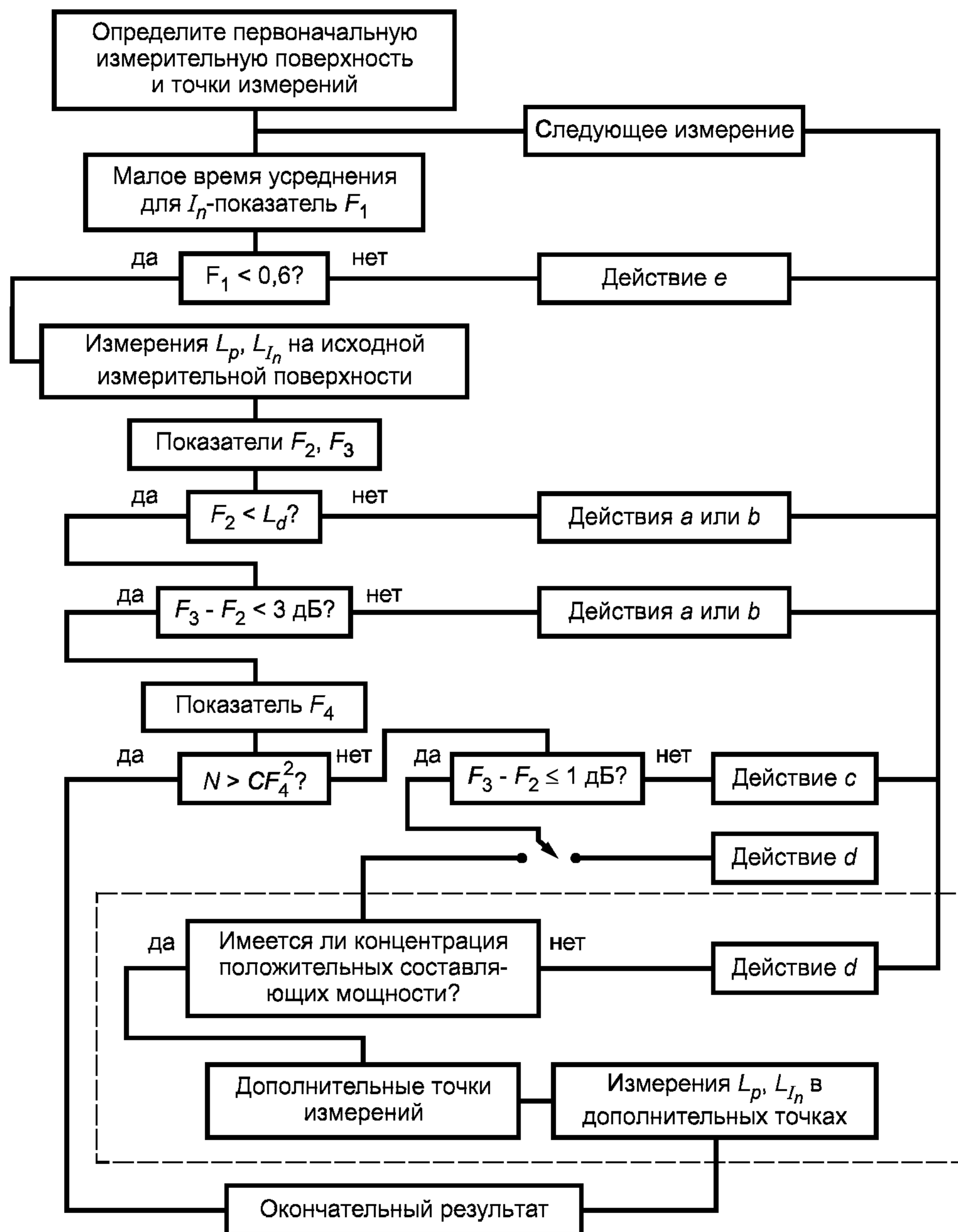
Рисунок Б.1 — Алгоритм достижения необходимой точности
