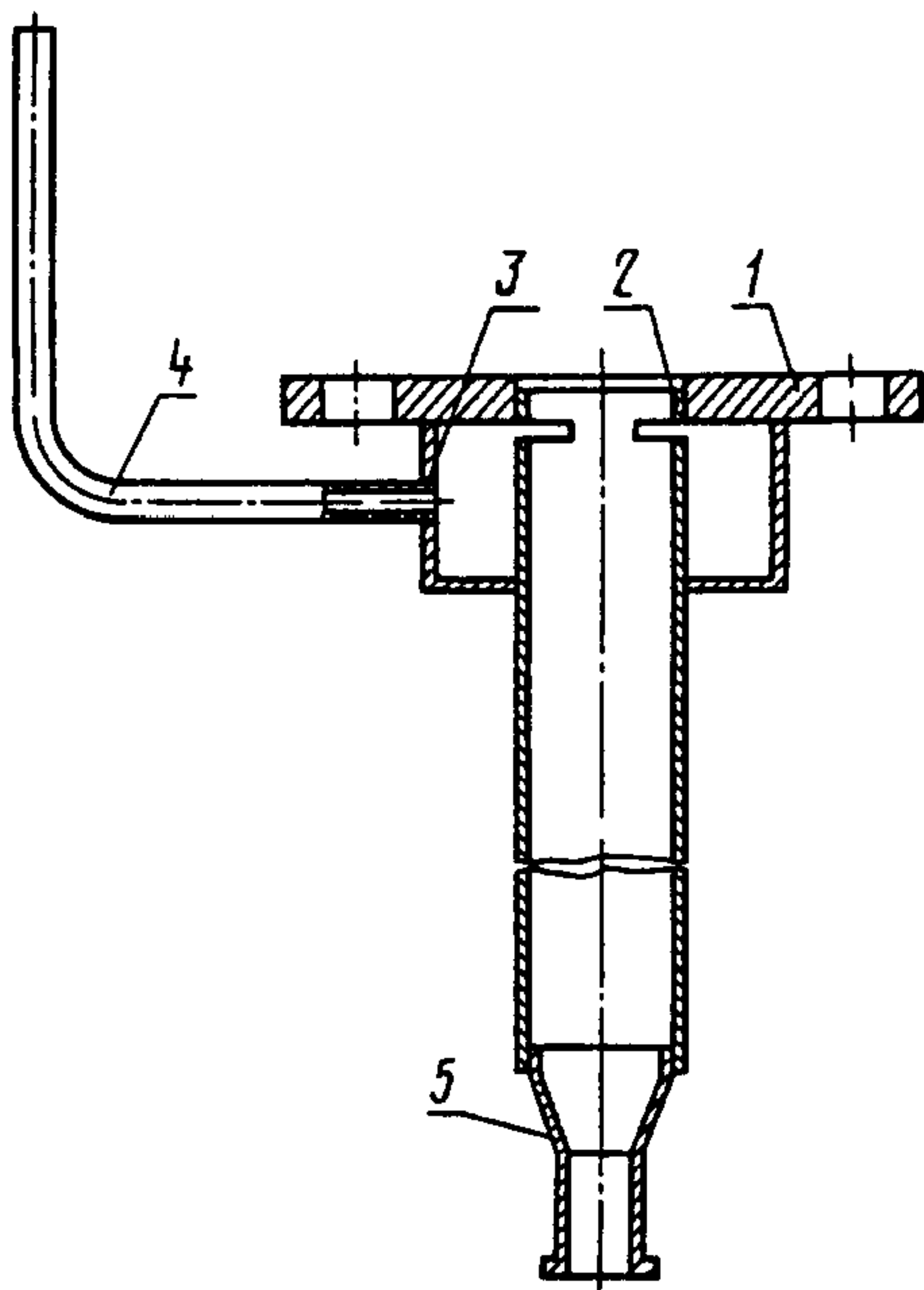
Схема входного штуцера
