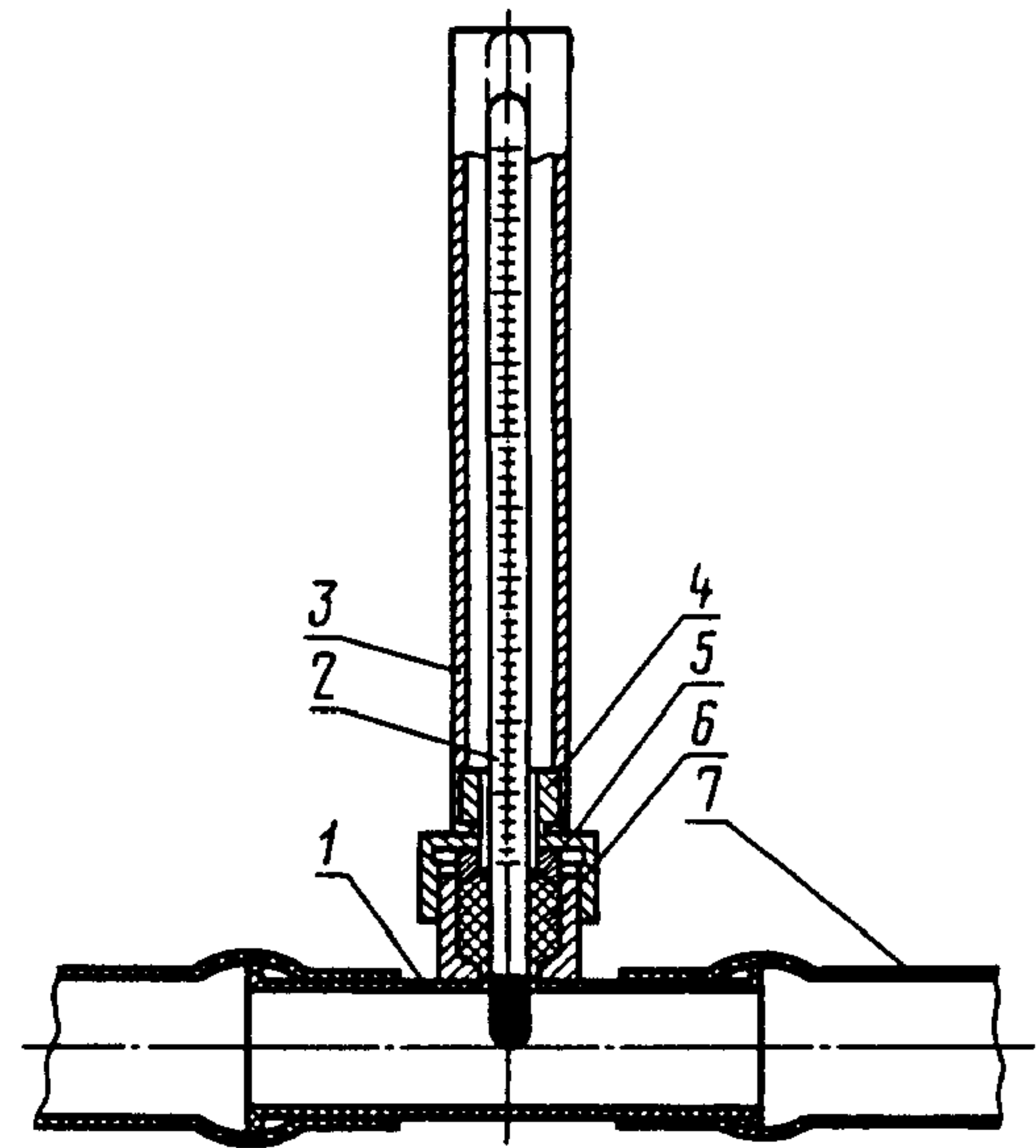
Схема установки термометра в линию
