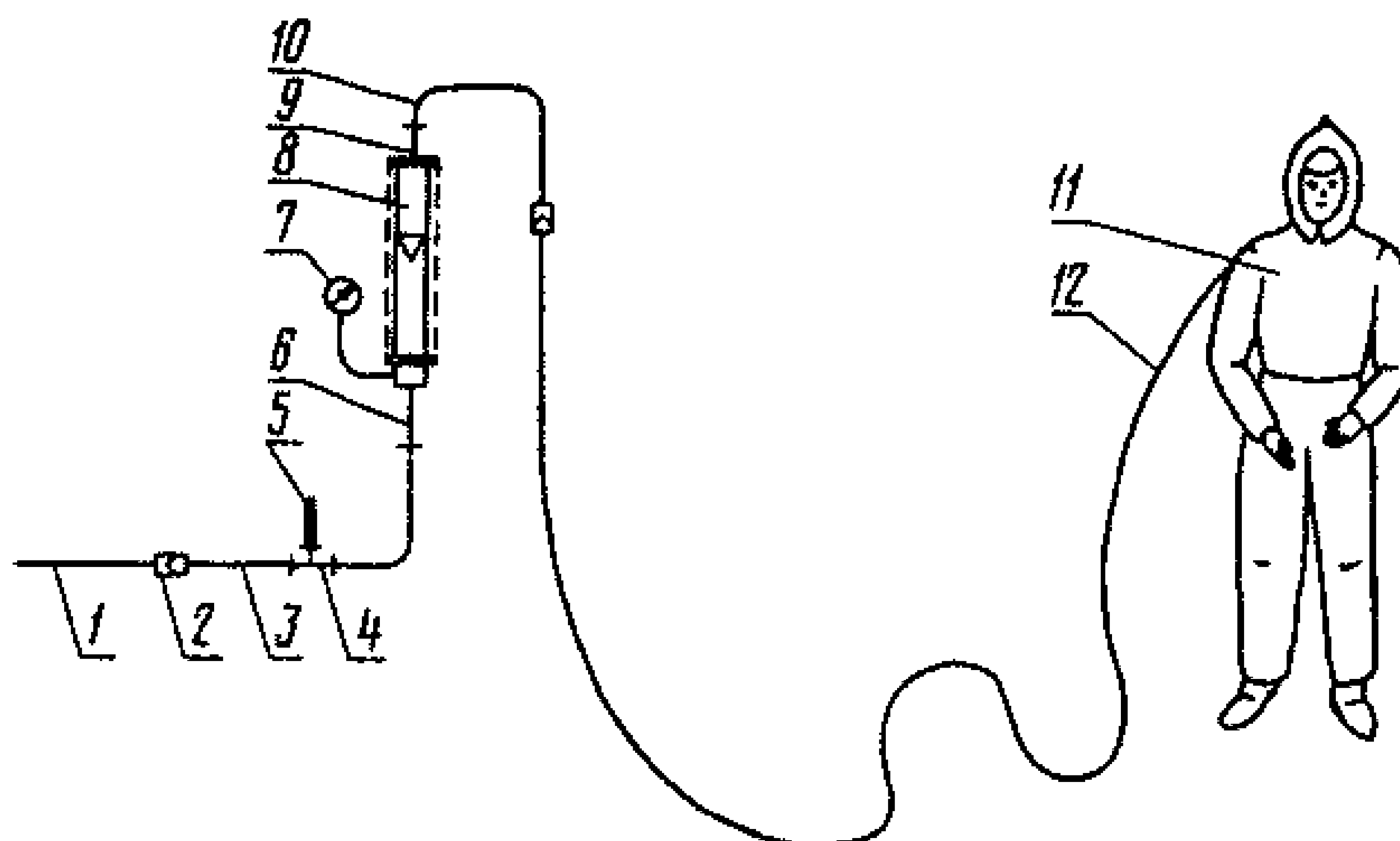
Схема установки ротаметра в технологическую линию
