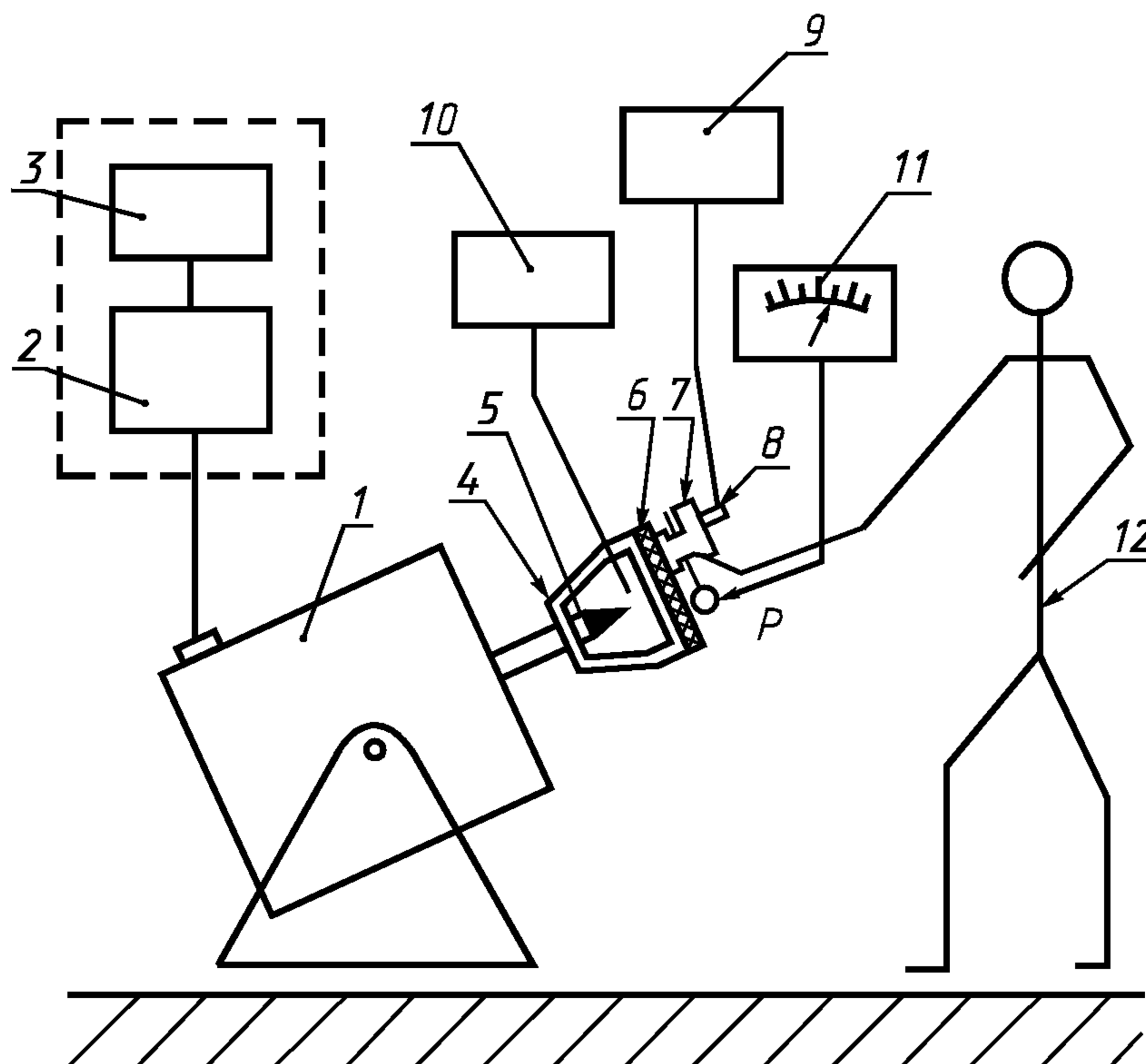
1 — вибростенд; 2 — усилитель мощности; 3 — генератор сигнала; 4 — рукоятка; 5 — контрольный вибропреобразователь; 6 — испытуемое изделие; 7 — адаптер; 8 — основной вибропреобразователь; 9 — виброметр для измерения эффективности; 10 — виброметр для контроля вибростенда; 11 — силоизмерительное устройство; 12 — оператор-испытатель (прикладывает усилие нажатия P )
