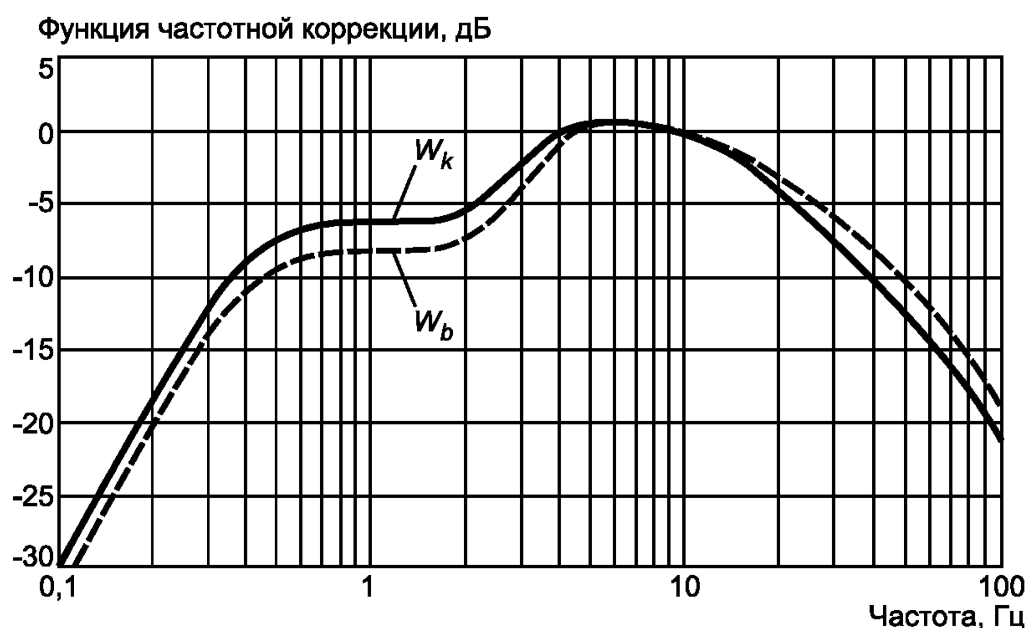
Рисунок 2 — Функции частотной коррекции W_b и W_k
