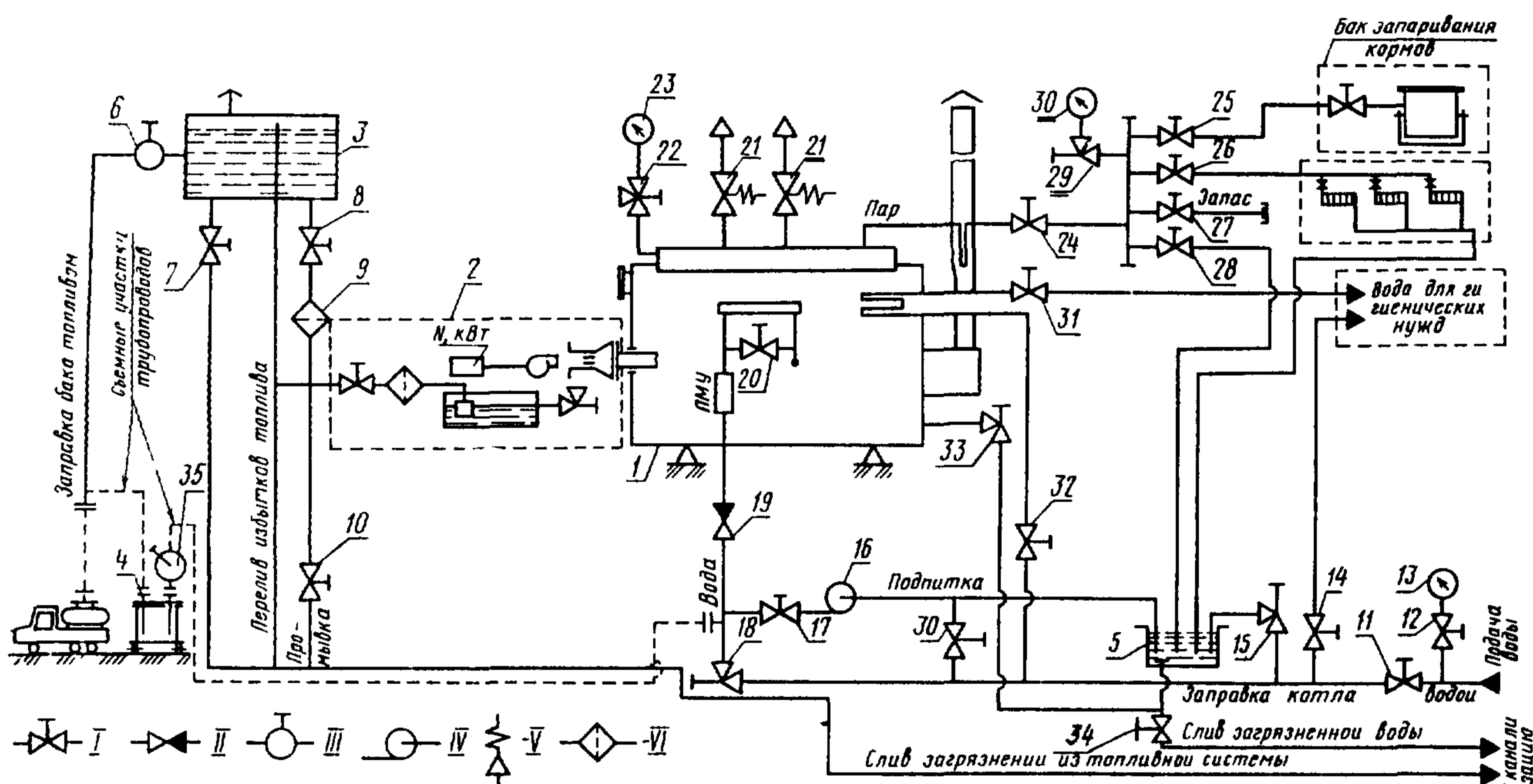
Схема котла КВ-300 М в сборе
