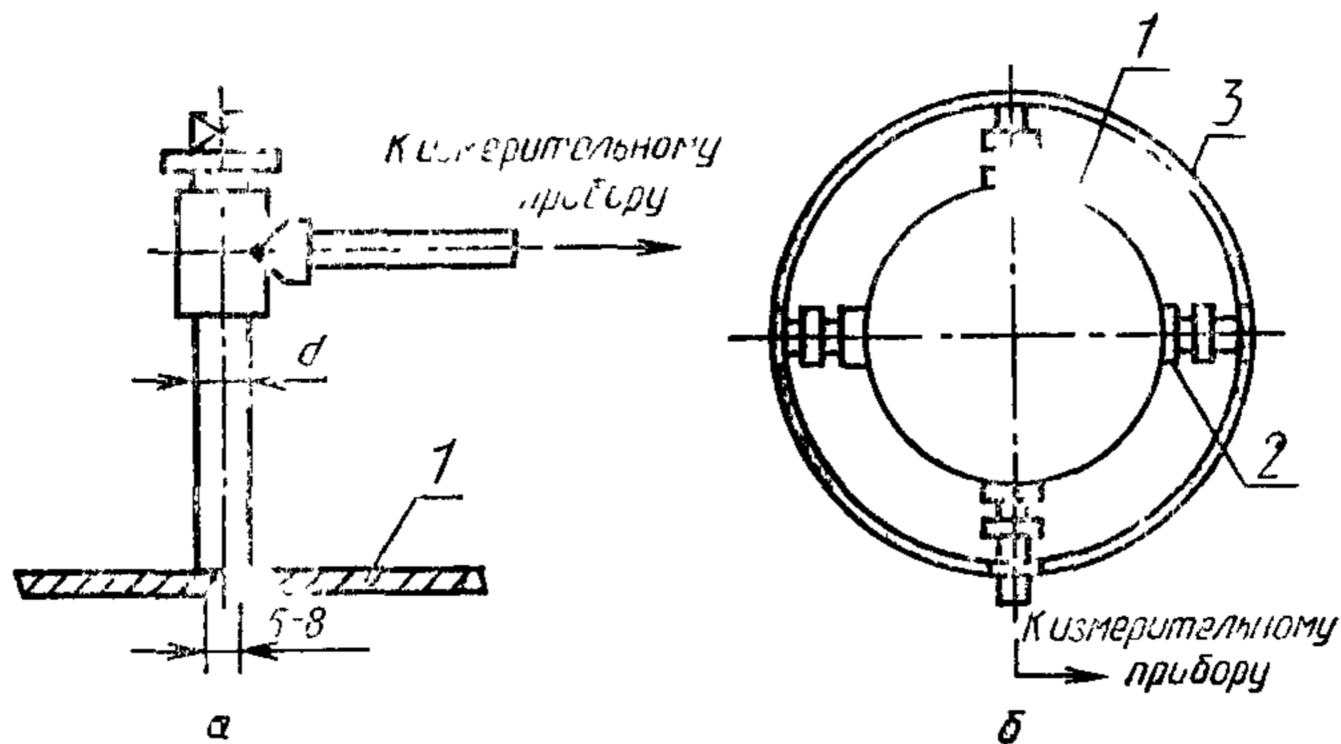
1 — стенка газохода; 2 — патрубок; 3 — соединительный трубопровод.
