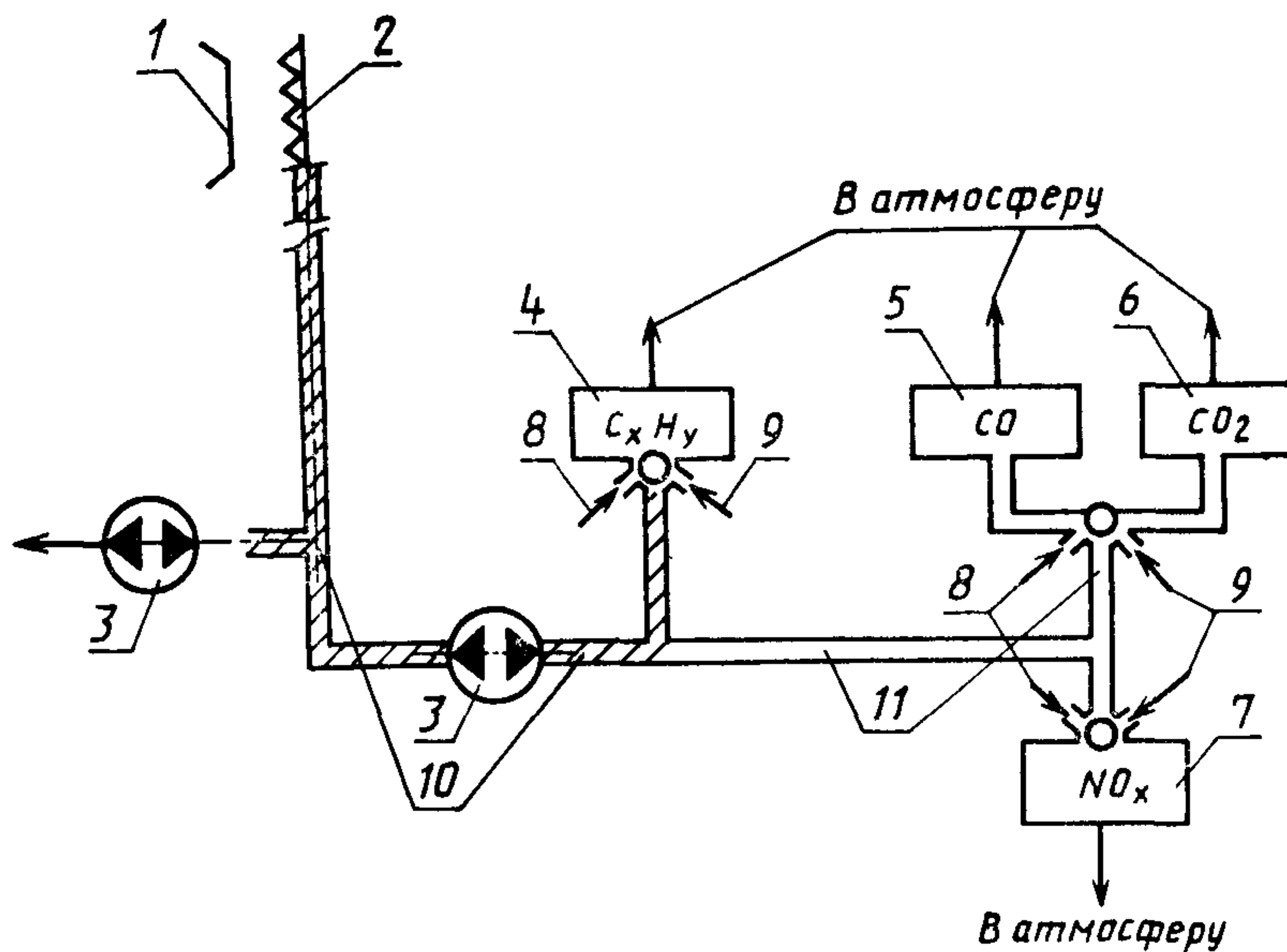
Схема системы отбора и анализа проб газа
