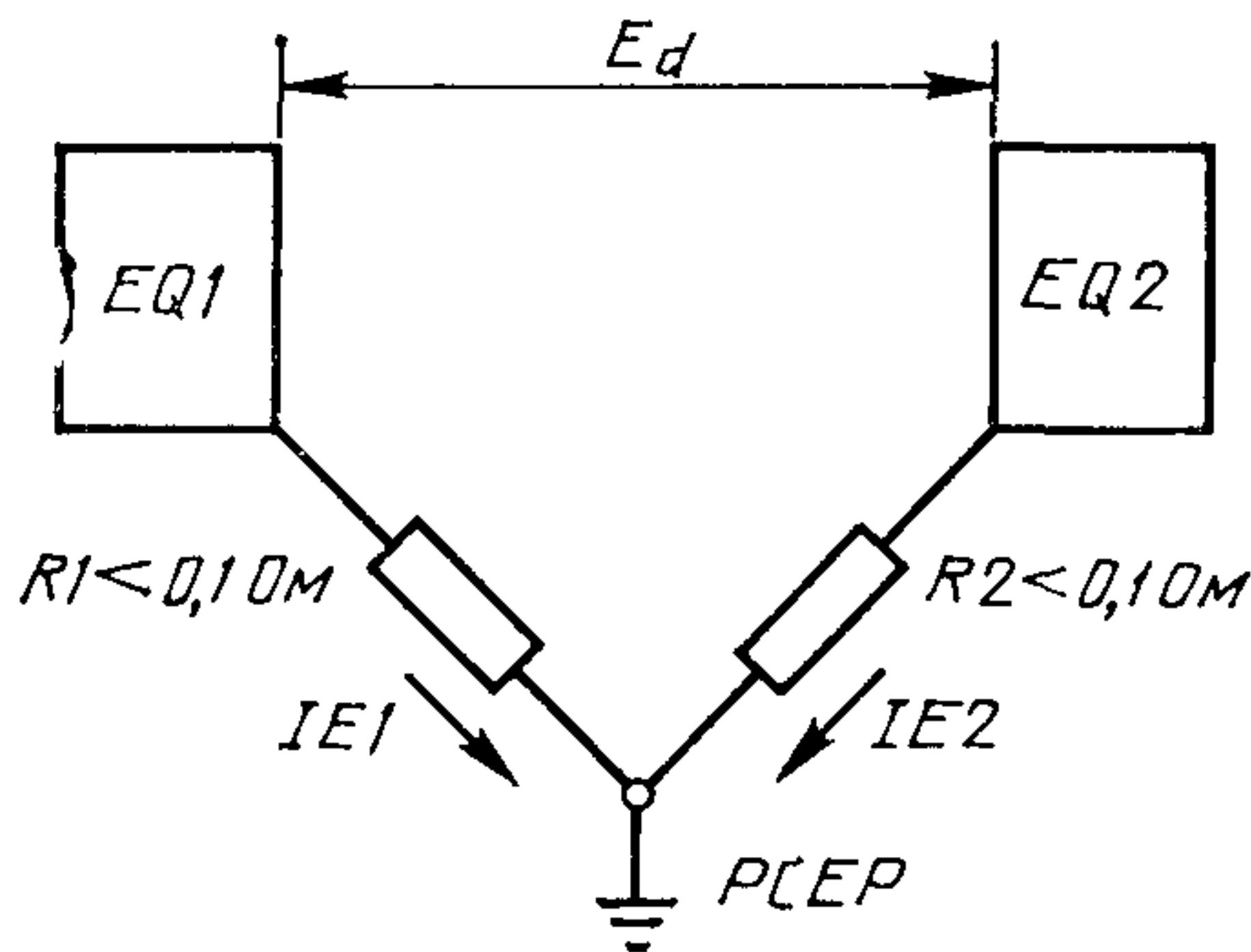
Рис. 4. Ток утечки на землю
