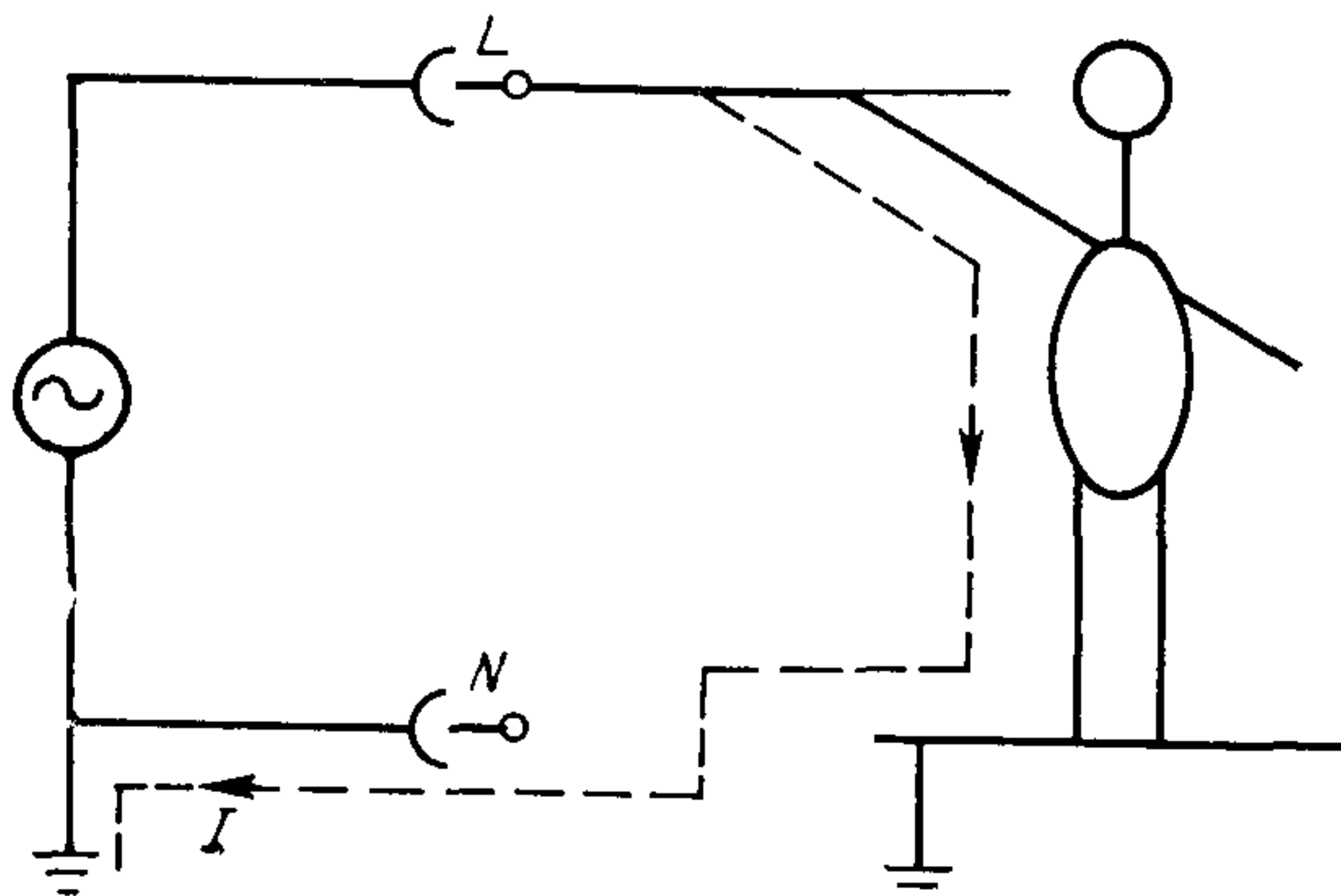
Рис. 1. Опасность, вызванная контактом с сетью
