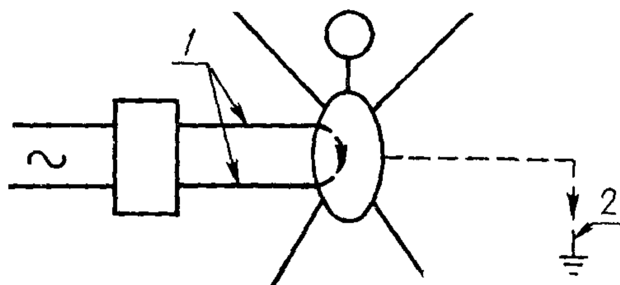
Рис 2. Ток утечки на пациента
