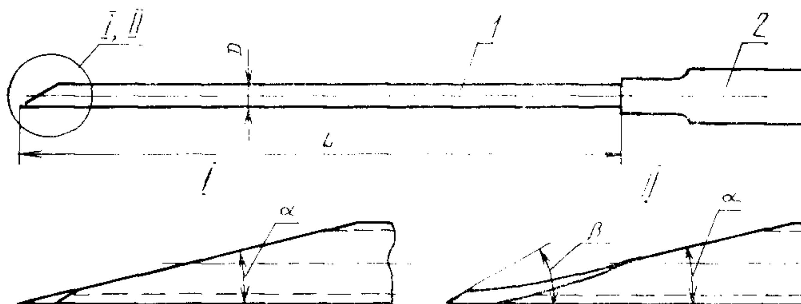
1—головка; 2—труба Черт. 1
