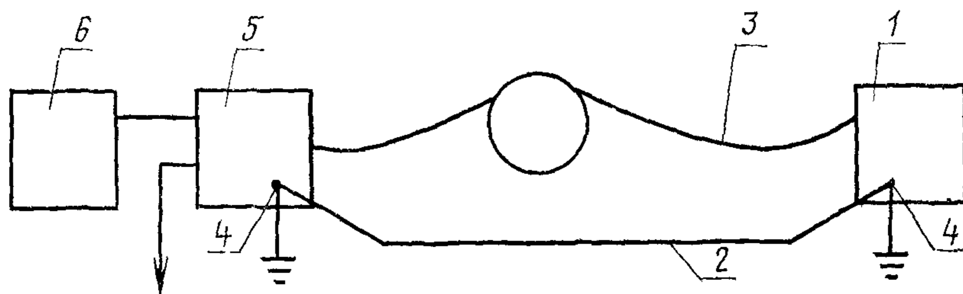
Расположение оборудования при измерении напряжения радиопомех
